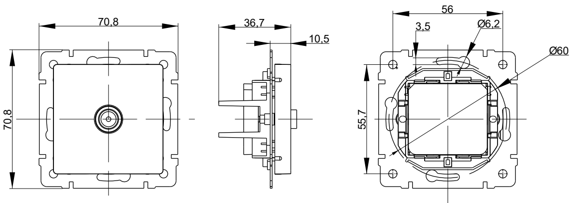
Телевизионная розетка
