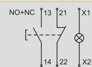
Электрическая схема
