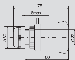
Габаритные размеры
