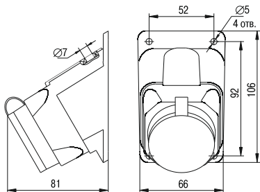
Рисунок 13 – Розетка с защитной крышкой угловая настенная РБУ13-1-0м
