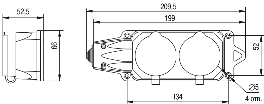
Рисунок 10 – Розетка (колодка) двухместная с защитными крышками РБ32-1-0м
