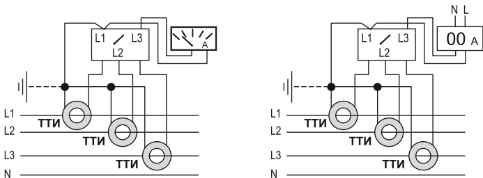
Рисунок 8. Подключение амперметров через трансформаторы тока 3-фазной сети с использованием селективного переключателя
