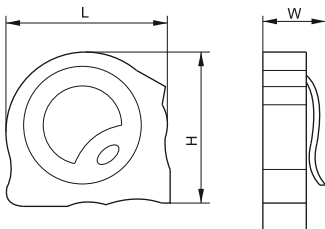
Рисунок 1 – Габаритные размеры рулеток
