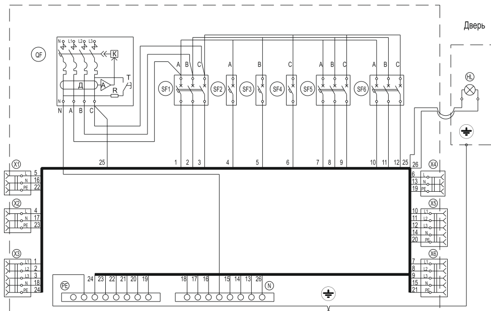
Рисунок 1 – Схема электрическая
