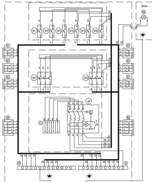
Рисунок 1 – Схема электрическая
