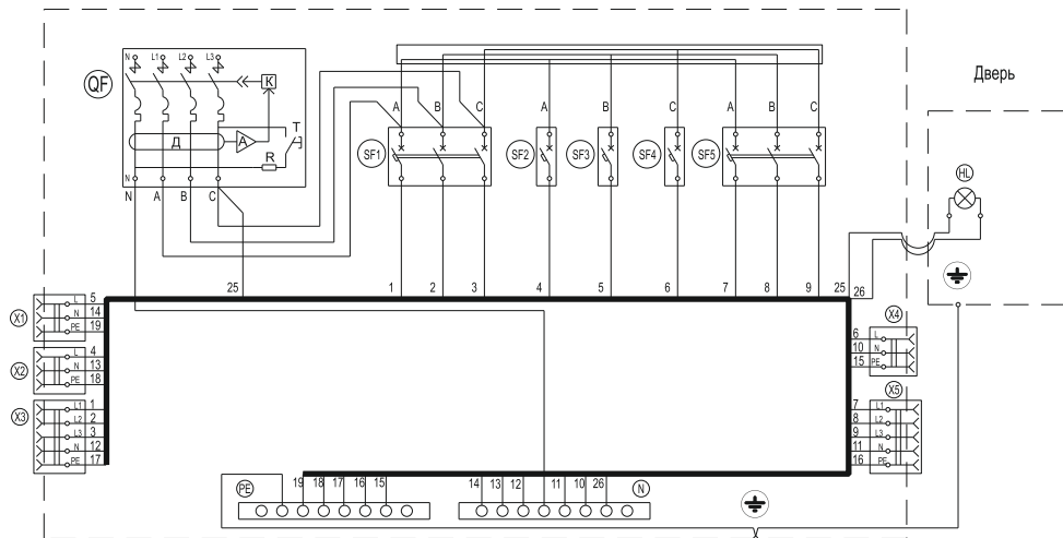
Рисунок 1 – Схема электрическая
