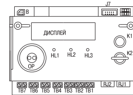
Рисунок 1 – Интерфейсы счетчика
