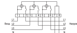
Рисунок А.2 – Схема прямого подключения счётчиков
