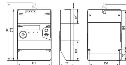
Рисунок А.1 – Габаритные и присоединительные размеры счётчиков
