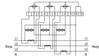
Рисунок А.4 – Схема подключения счётчиков через трансформаторы тока и напряжения
