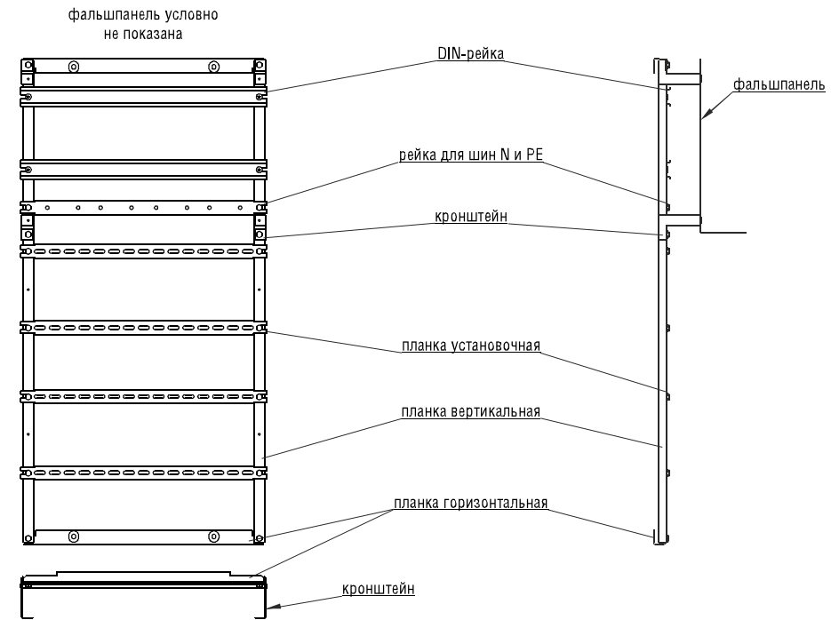
Компоновочная схема щита
