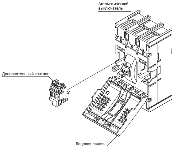
Рисунок 3 – Установка устройств в выключатели BA88 серии MASTER на примере левостороннего исполнения
