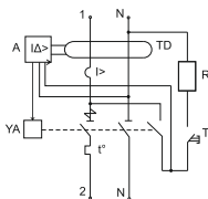
Рисунок А.2 – Схема электрическая принципиальная АВДТ тип АС/ Figure A.2 – Electric schematic diagram of AVDT of AC type
