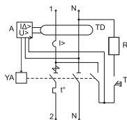
Рисунок А.3 – Схема электрическая принципиальная АВДТ тип А/ Figure A.3 – Electric schematic diagram of AVDT of A type
