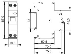
*предельное отклонение габаритных размеров \pm 0,5 мм/ deviation limit of dimensions is \pm 0,5 mm
