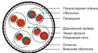
Рисунок 2 – Конструкция кабеля типа S/FTP
