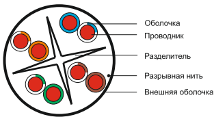
Рисунок 1 – Конструкция кабеля типа U/UTP
