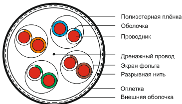
Рисунок 1 – Конструкция кабеля типа S/FTP
