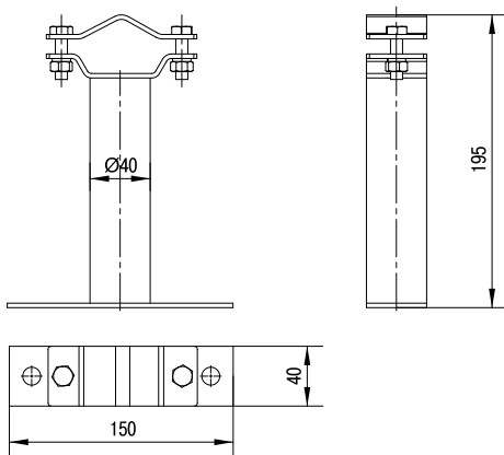
Рисунок 1 – Габаритные размеры
