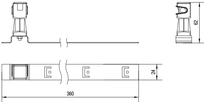
Рисунок 1 – Габаритные размеры
