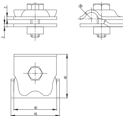
Рисунок 1 – Габаритные размеры
