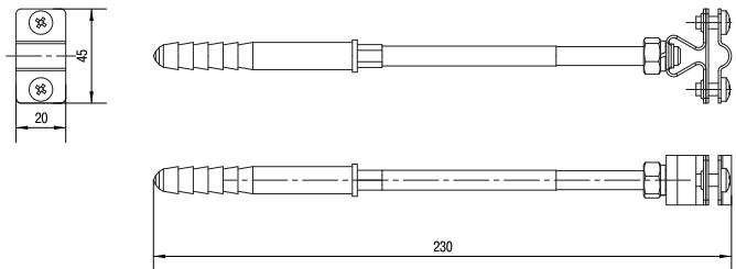
Рисунок 1 – Габаритные размеры
