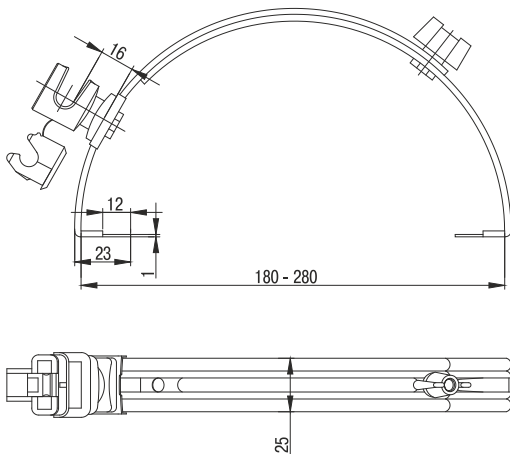
Рисунок 1 – Габаритные размеры
