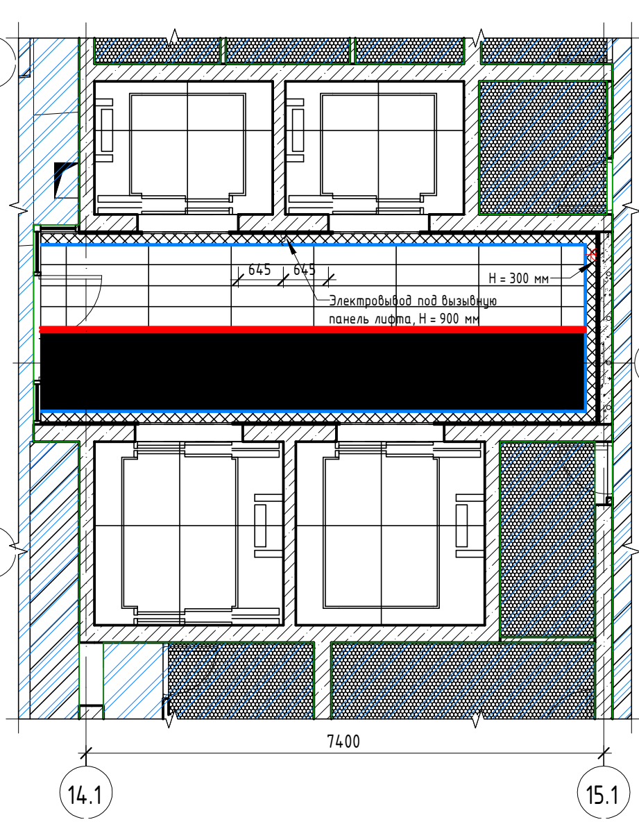
План расстановки выключателей осветительных приборов по группам -2 этаж. (1 : 75)
