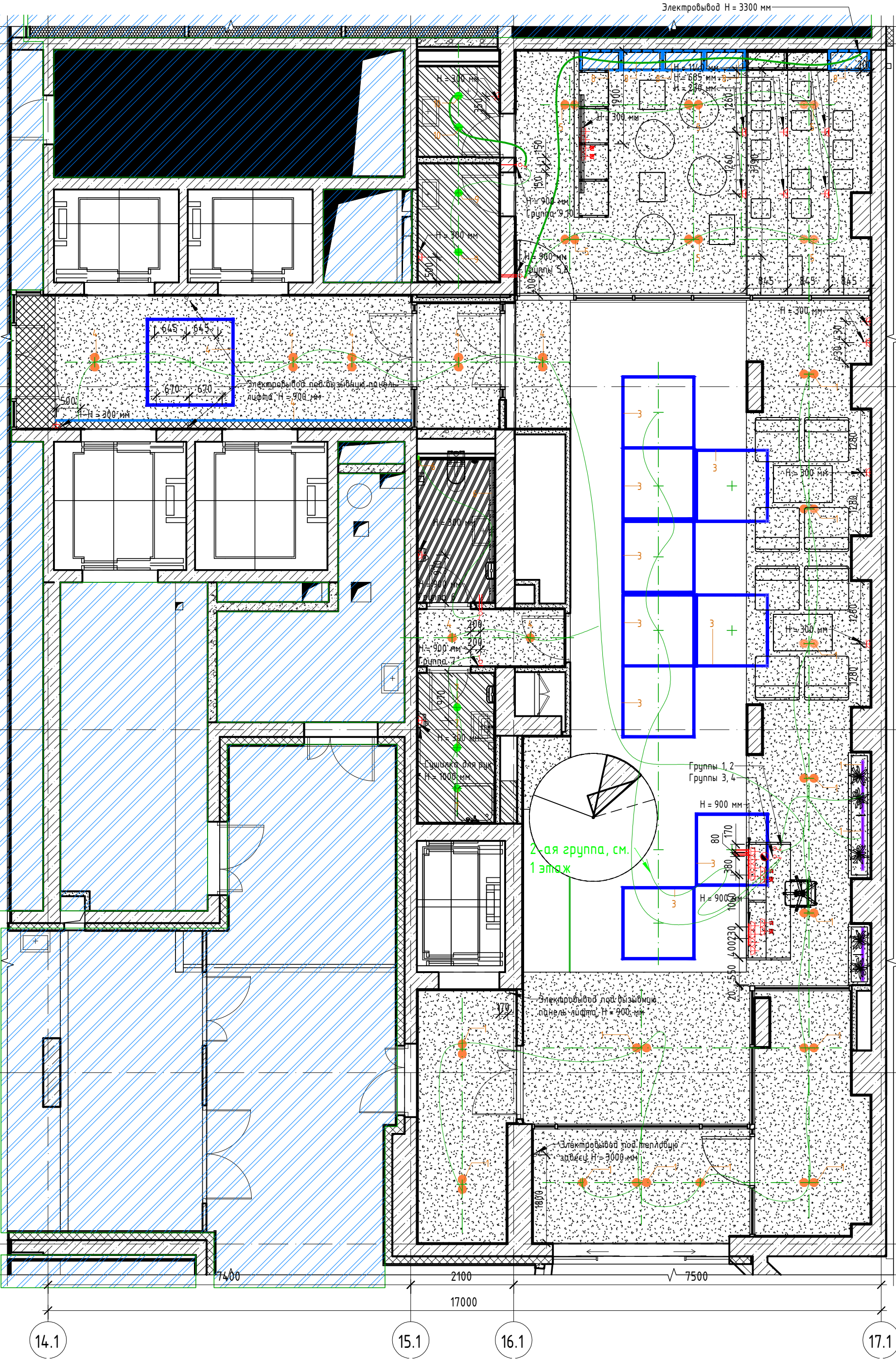
План расстановки выключателей осветительных приборов по группам -1 этаж. (1 : 75)
