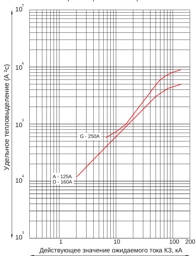
МССВ габ. А - 125А, D - 160А кривая ограничения энергии
