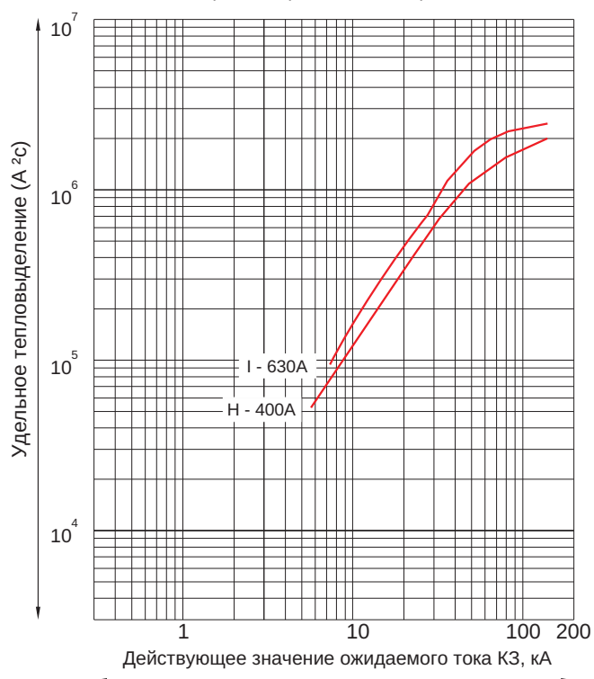
МССВ габ. Н - 400А, I - 630А кривая ограничения энергии
