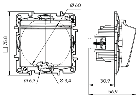
Выключатель карточный
