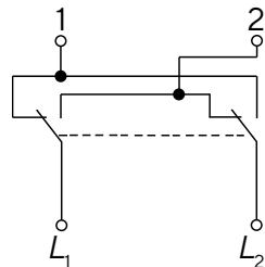
Переключатель двухклавишный перекрестный
