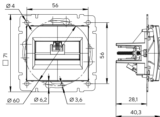
Розетка телефонная
