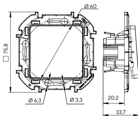
Выключатель двухклавишный
