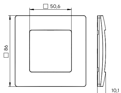
Рамка одноместная
