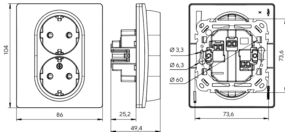
Розетка двухместная с заземлением с защитными шторками в сборе
