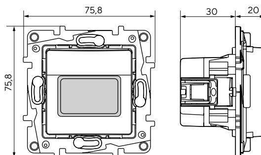
Датчик движения
