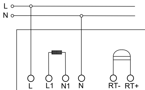
Термостат электронный
