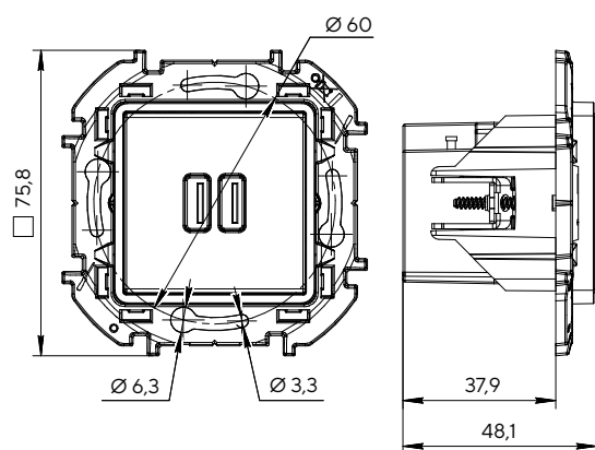
Розетка USB A + A
