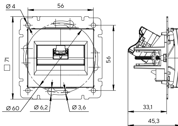
Розетка компьютерная одноместная
