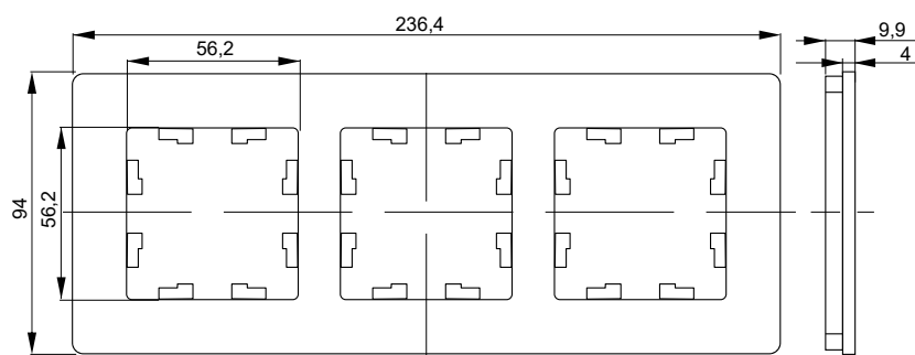
Рамка трехместная
