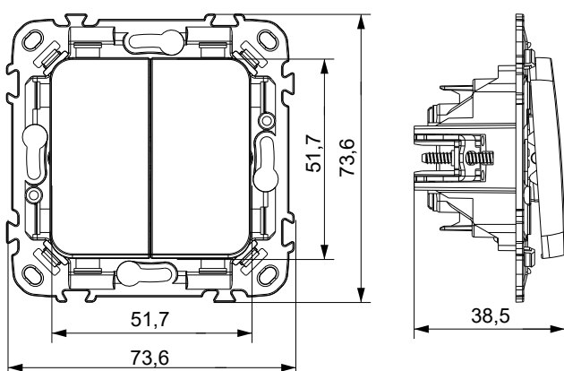
Выключатель двухклавишный, выключатель двухклавишный кнопочный, переключатель двухклавишный
