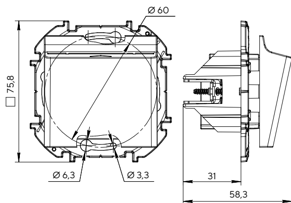
Выключатель карточный
