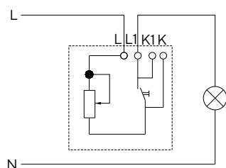
Светорегулятор
