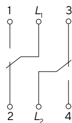
Переключатель двухклавишный самовозвратный
