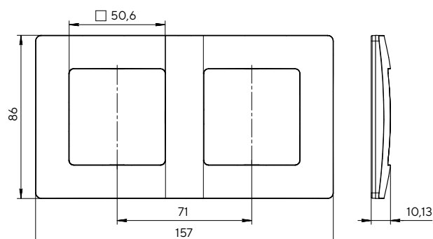
Рамка двухместная
