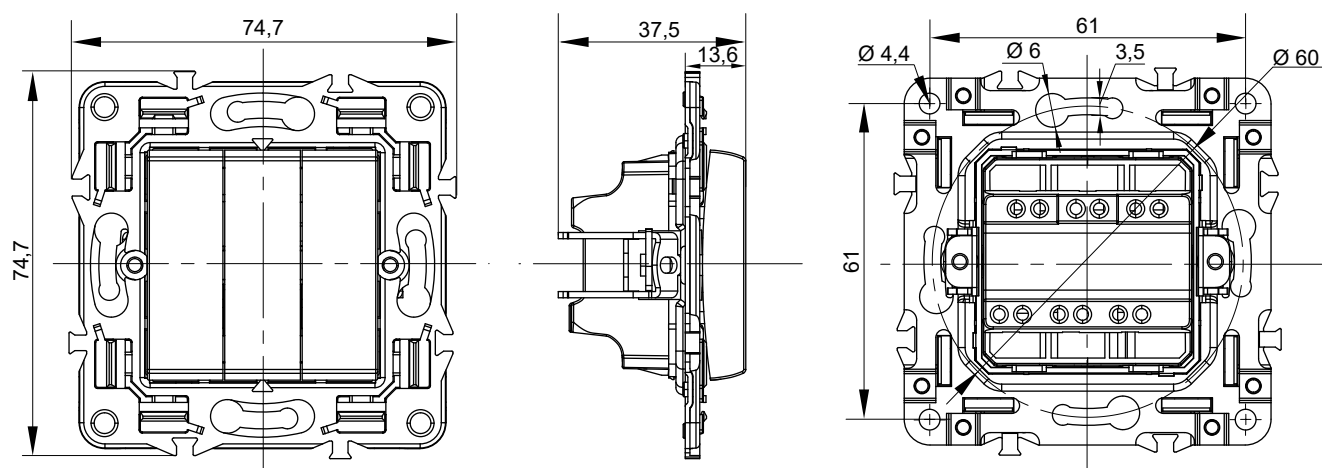
Выключатель трехклавишный
