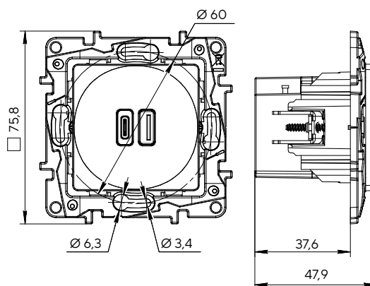
Розетка USB A + C
