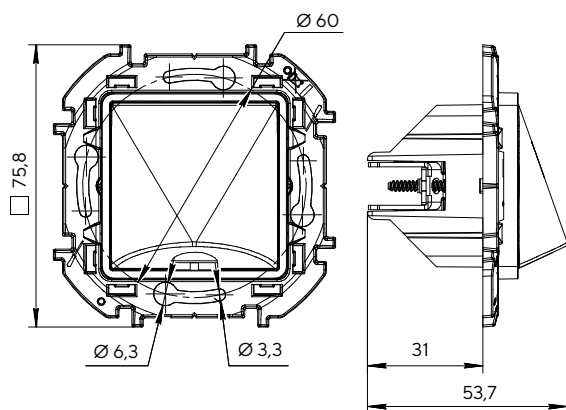
Вывод кабеля с зажимом для кабеля
