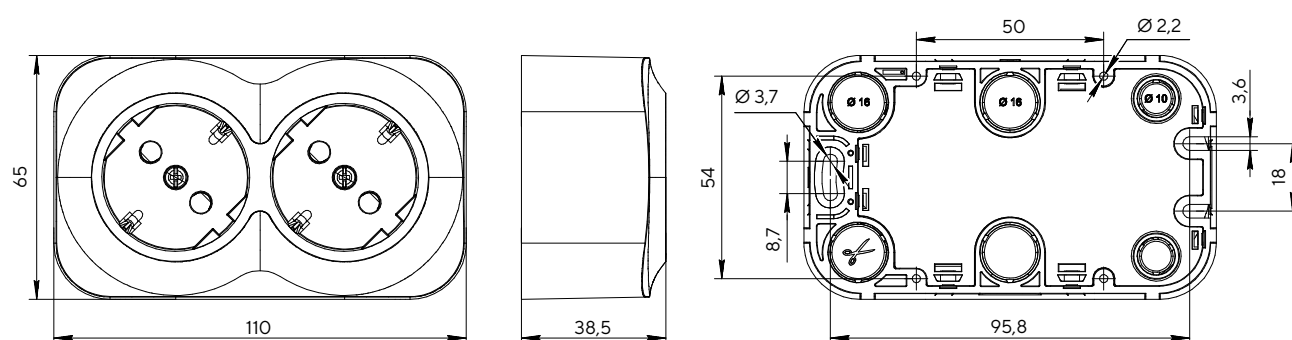
Розетка двухместная с заземлением с защитными шторками
