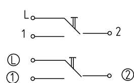
Переключатель двухклавишный кнопочный
