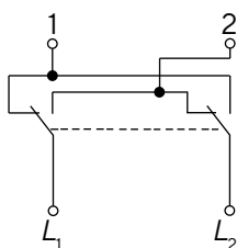
Переключатель одноклавишный перекрестный
