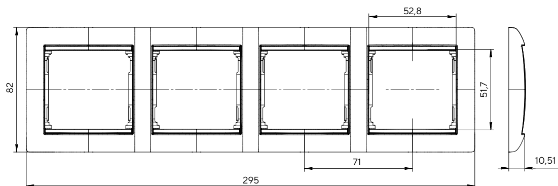
Рамка четырехместная
