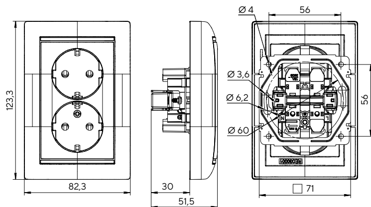
Розетка двухместная с заземлением и защитными шторками
