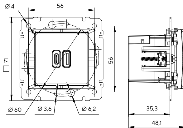
Розетка USB A + C
