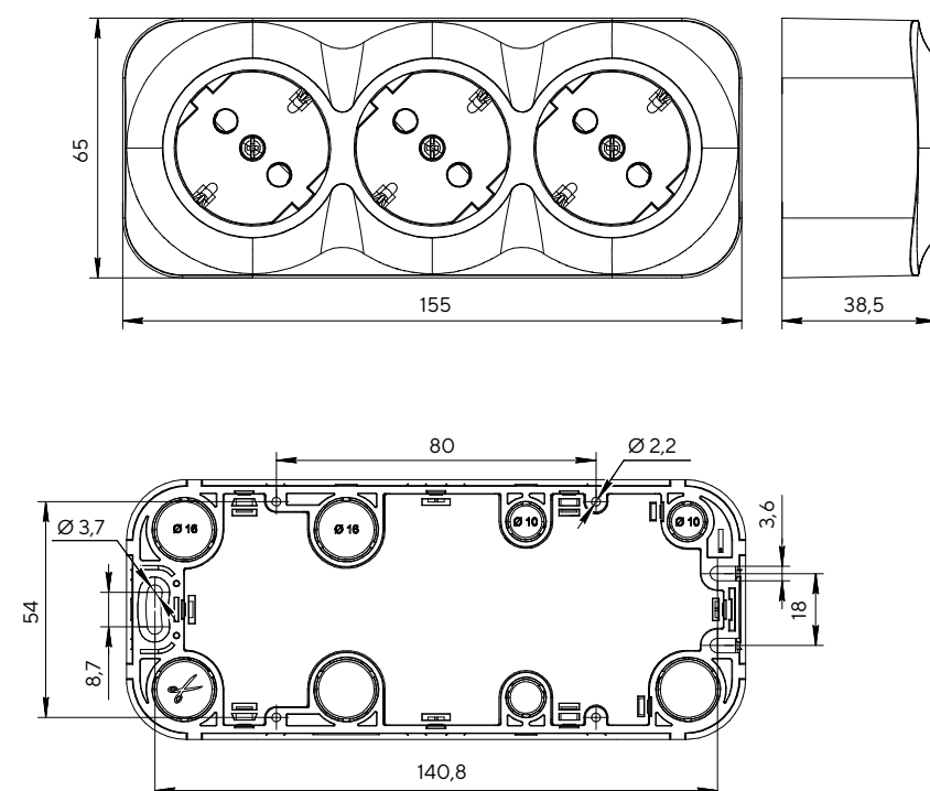
Розетка трехместная с заземлением с защитными шторками
