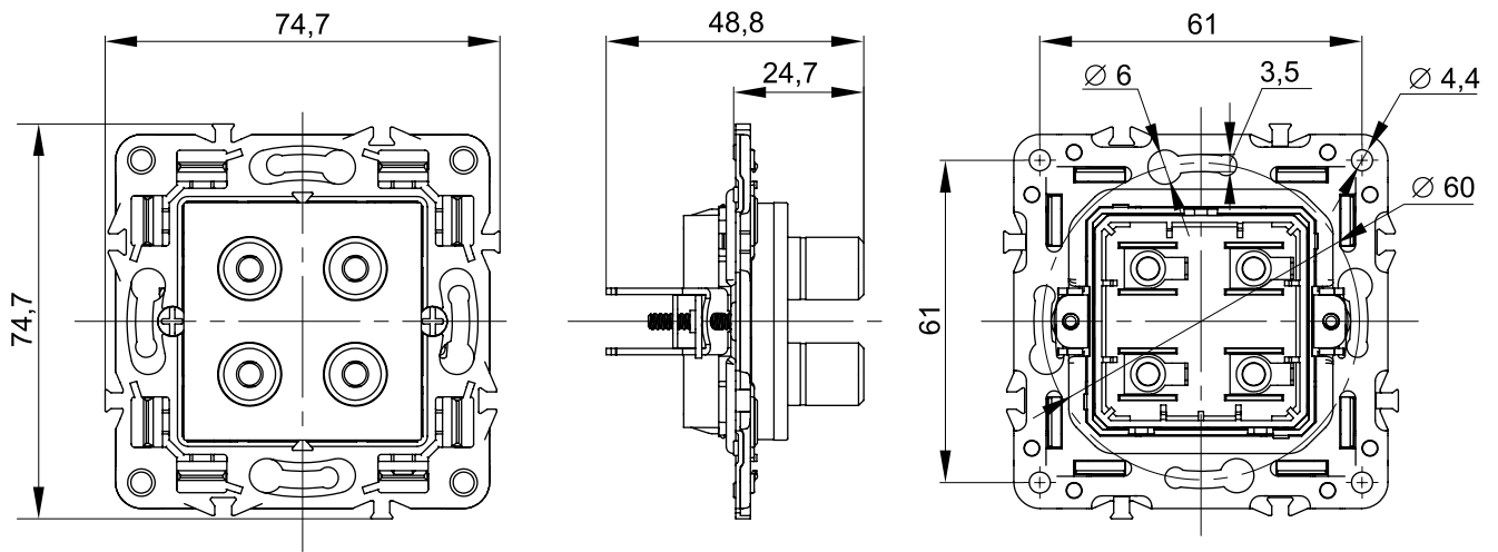
Розетка акустическая
