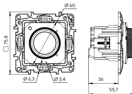
Термостат
