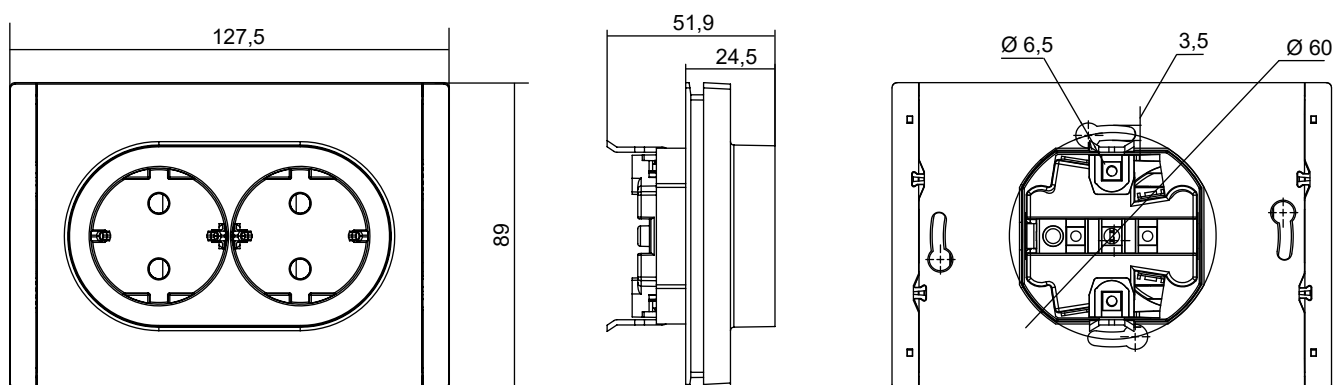
Розетка двухместная, I_n = 16\text{ A}
