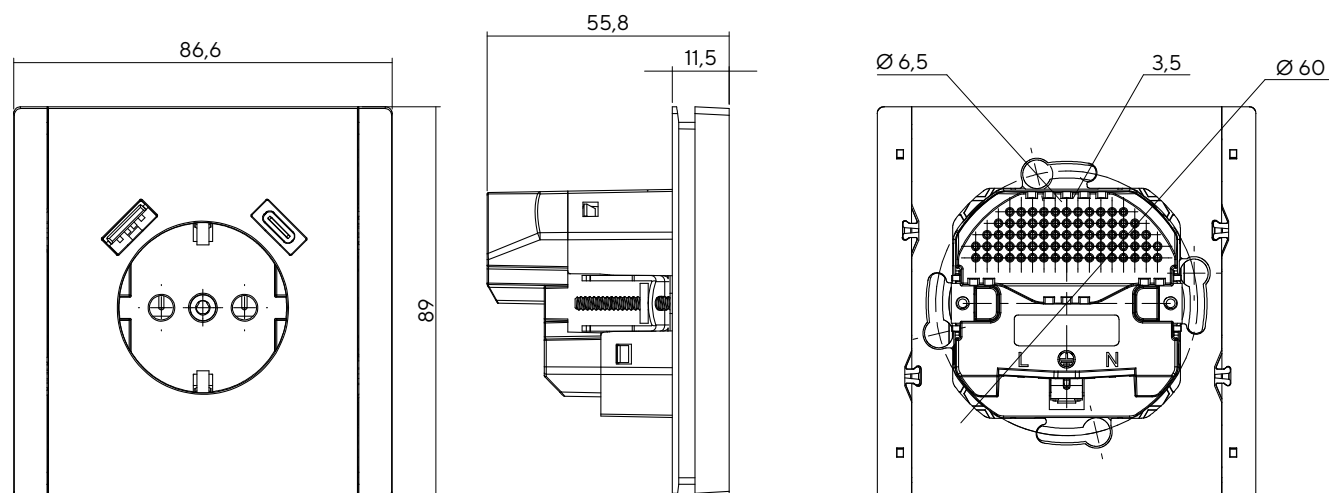
Розетка одноместная с USB-разъемами А + С
