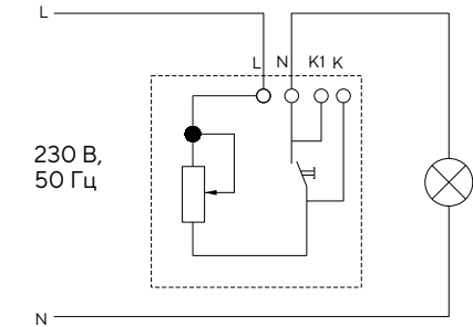
Светорегулятор
