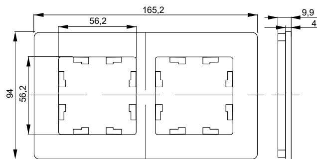
Рамка двухместная
