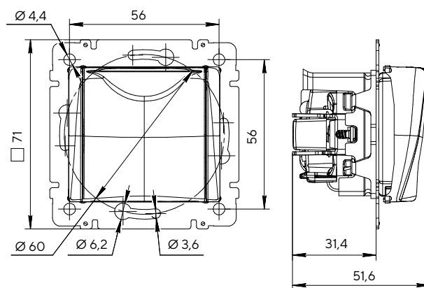
Розетка одноместная с заземлением с защитными шторками и крышкой
