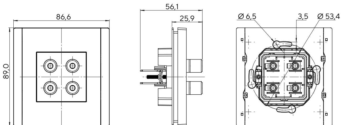
Аудиорозетка
