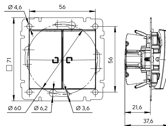
Выключатель/переключатель двухклавишный с подсветкой
