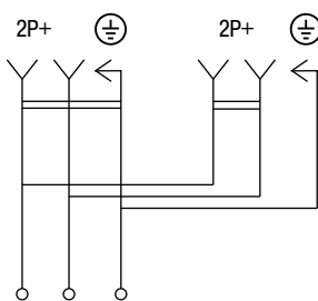
Розетка двухместная с заземлением
