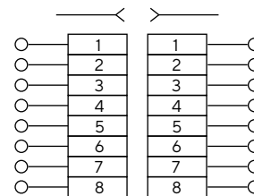
Розетка компьютерная двухместная
