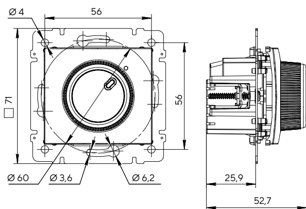
Светорегулятор
