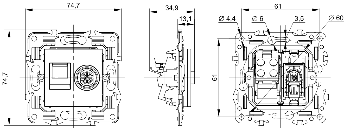
Розетка двухместная TV + компьютерная RJ45
