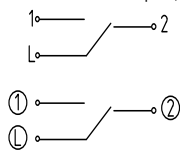
Переключатель двухклавишный
