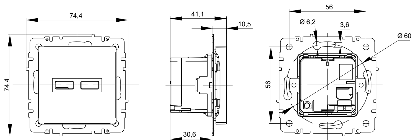
Розетка USB A + A
