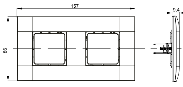
Рамка двухместная
