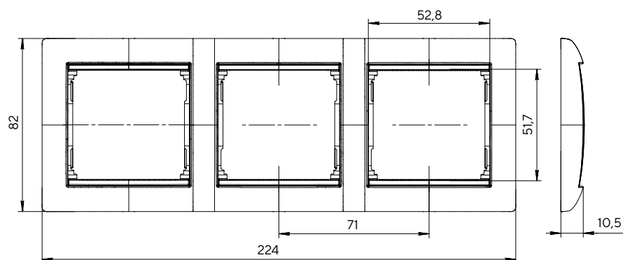
Рамка трехместная
