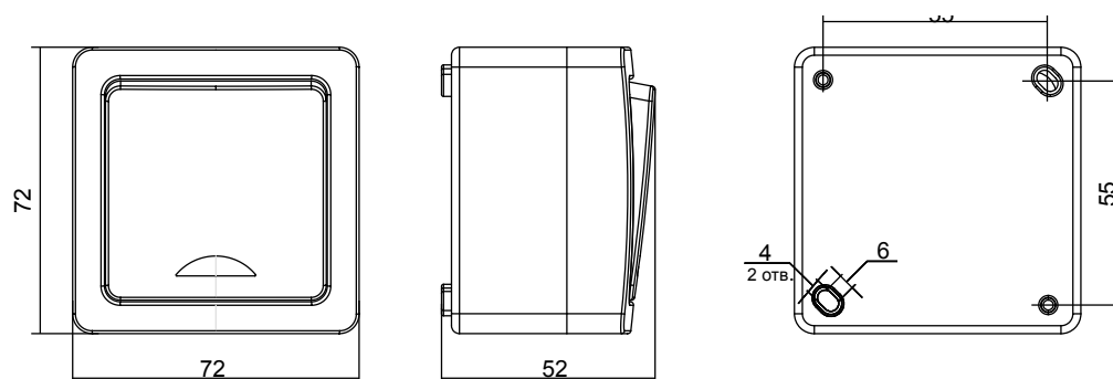
Выключатель одноклавишный с индикацией
