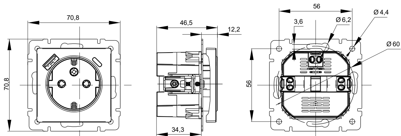
Розетка силовая + 2 USB A + C
