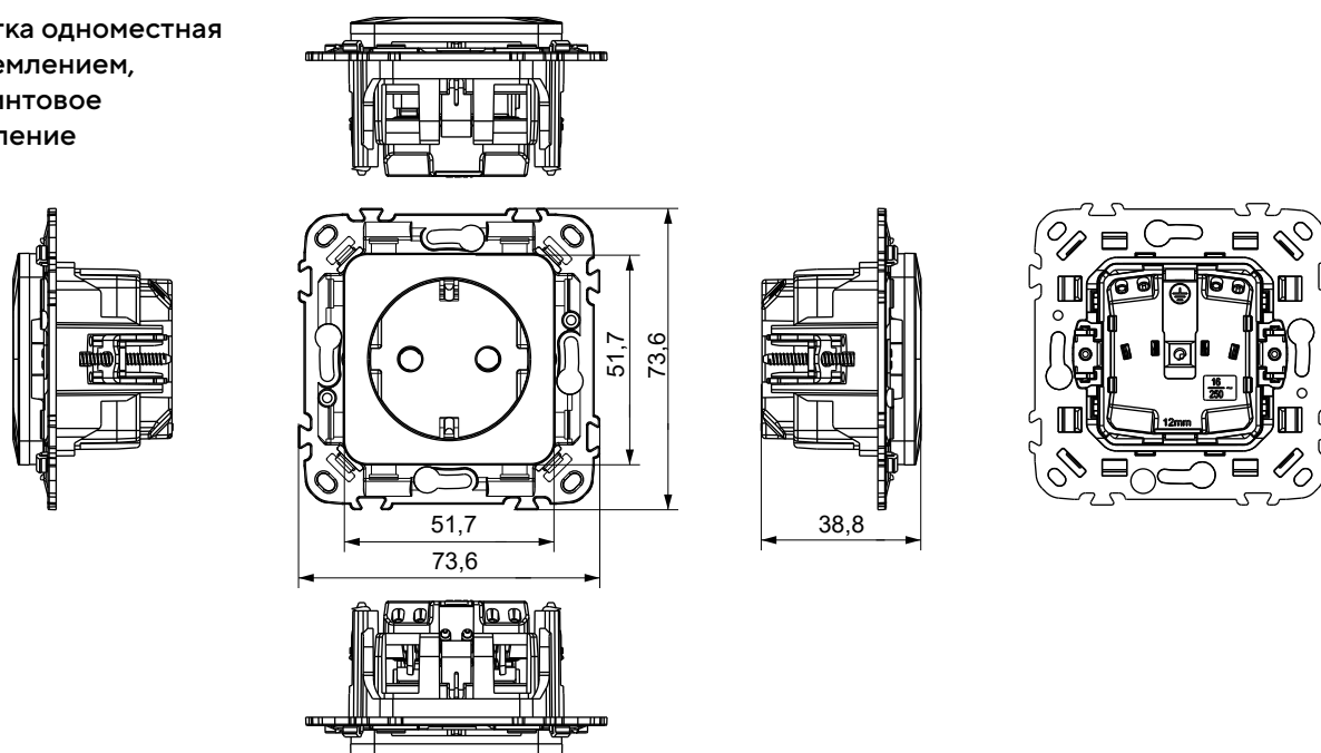
Розетка одностная с заземлением, винтовое крепление
