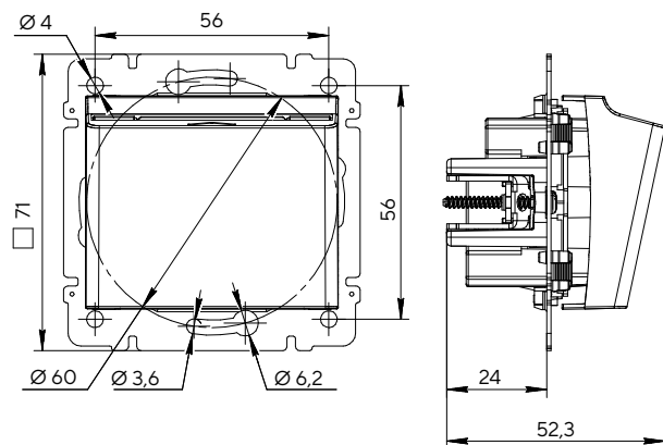
Выключатель карточный
