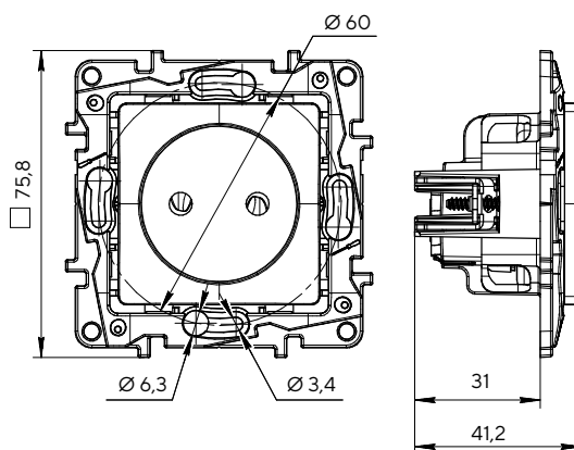
Розетка одноместная с заземлением с защитными шторками
