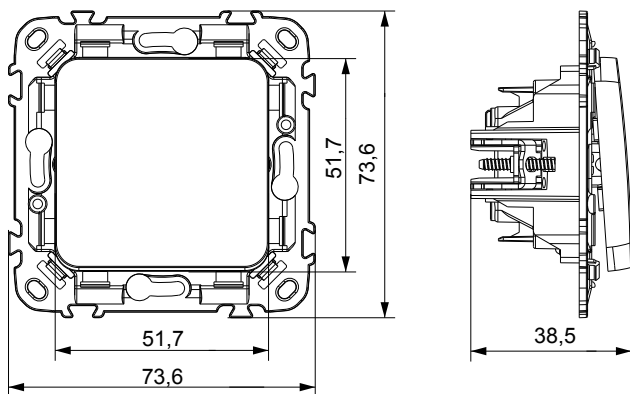
Выключатель одноклавишный, выключатель одноклавишный кнопочный, переключатель одноклавишный
