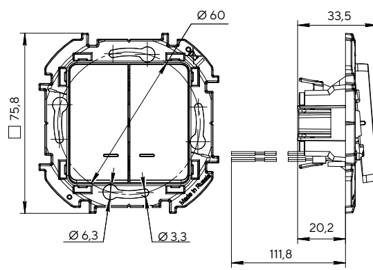
Выключатель двухклавишный с подсветкой/индикацией
