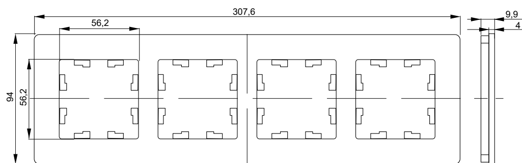
Рамка четырехместная
