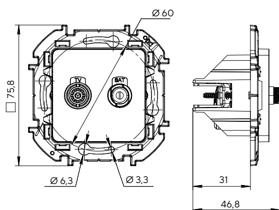
Розетка двухместная TV + SAT, тип «звезда»
