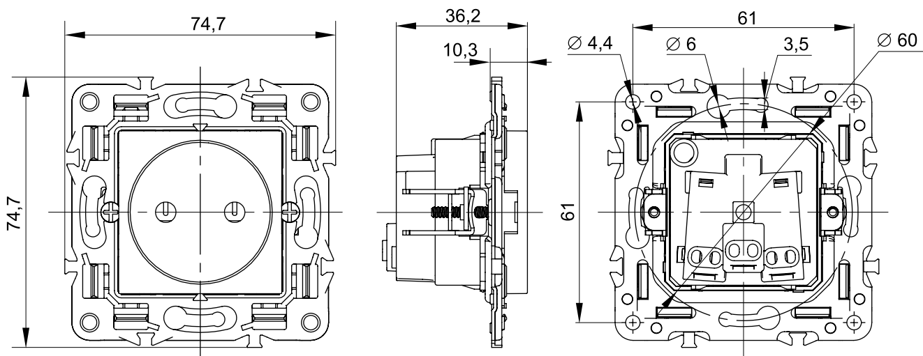
Розетка одноместная без заземления
