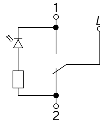
Переключатель одноклавишный проходной с индикацией
