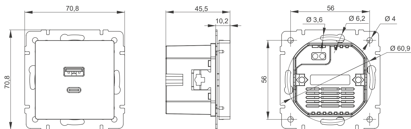
Розетка USB A + C 45 Вт
