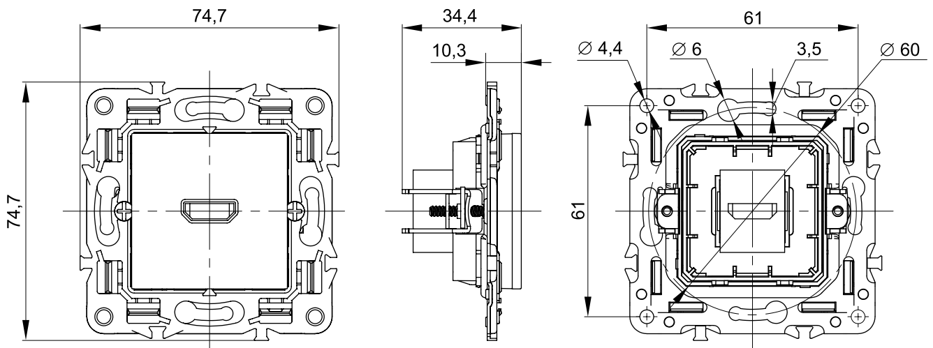
Розетка HDMI
