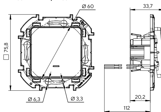
Выключатель одноклавишный с подсветкой/индикацией
