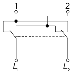
Переключатель одноклавишный перекрестный
