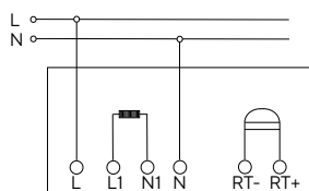
Терморегулятор
