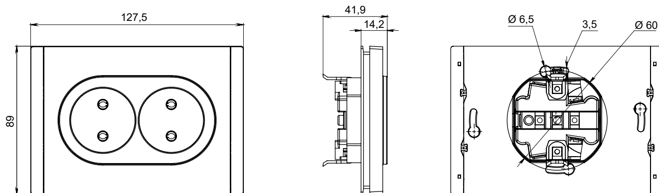
Розетка двухместная, I_n = 10\text{ A}
