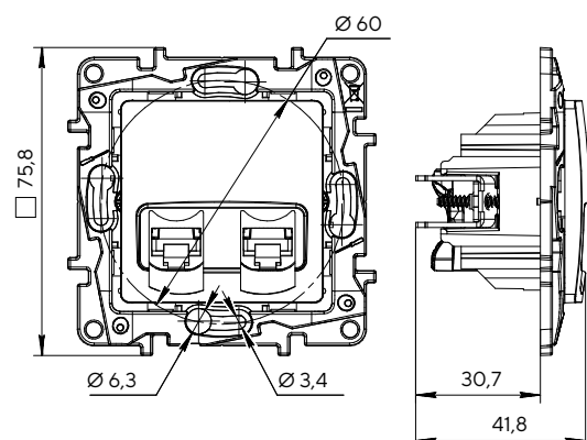
Розетка компьютерная двухместная RJ45
