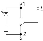
Переключатель одноклавишный проходной с индикацией
