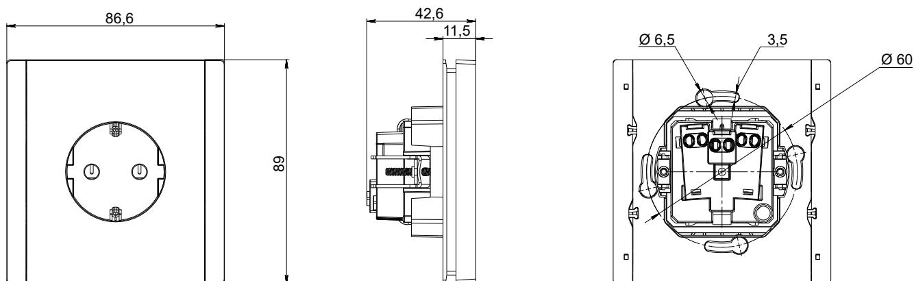
Розетка одностная, I_n = 16\text{ A}
