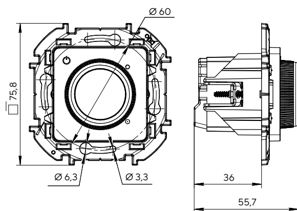
Термостат электронный с индикацией
