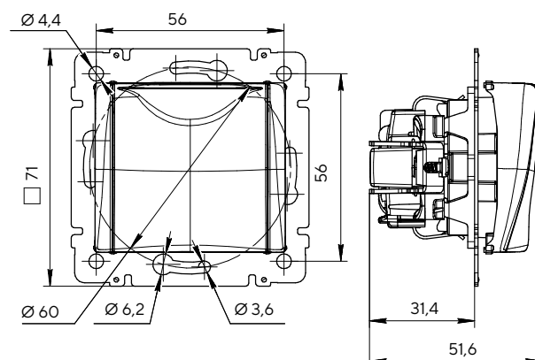
Розетка одностная с заземлением, защитными шторками и крышкой
