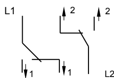
Выключатель двухклавишный проходной
