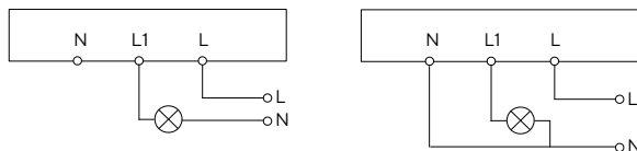
Светорегулятор
