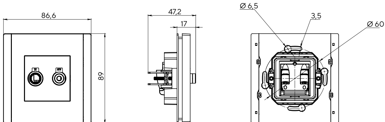
Розетка компьютерная RJ45 двухместная
