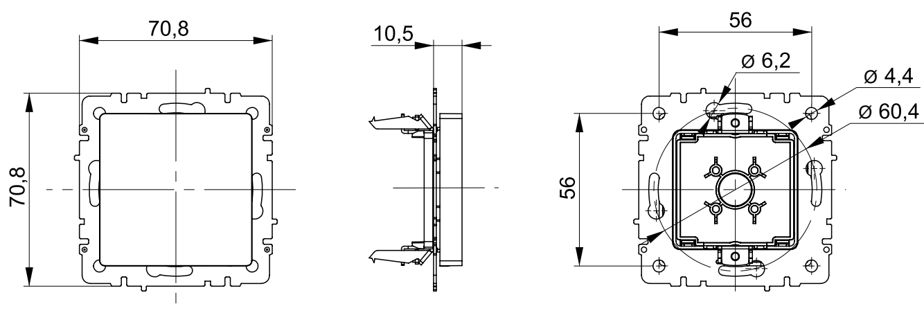
Заглушка встраиваемая
