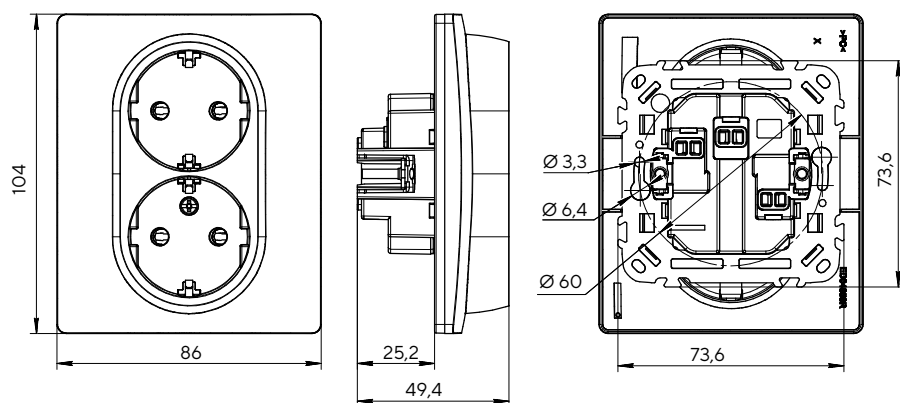
Розетка двухместная с заземлением с защитными шторками в сборе
