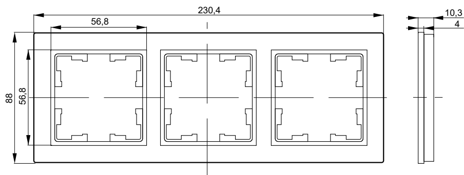
Рамка трехместная
