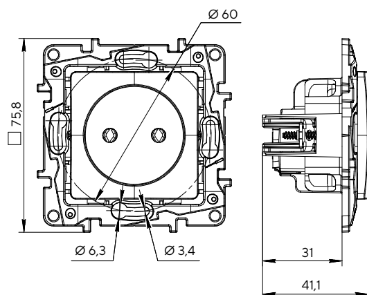
Розетка одноместная с заземлением без защитных шторок
