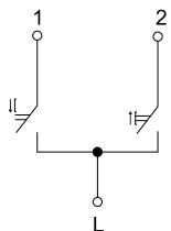
Кнопка вызова персонала с индикацией отдельная и выключатель двухклавишный с индикацией отдельный
