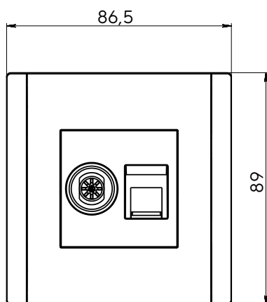
Розетка двухместная TV + компьютерная RJ45
