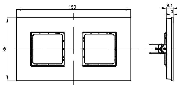
Рамка двухместная
