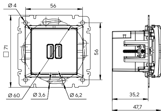
Розетка USB A + A
