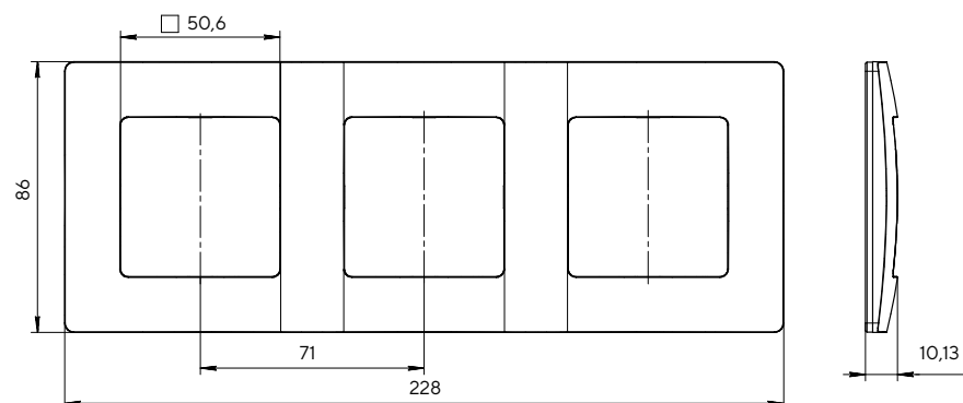
Рамка трехместная
