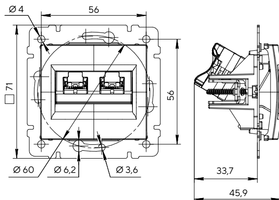
Розетка компьютерная двухместная
