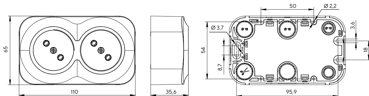
Розетка двухместная без заземления без защитных шторок
