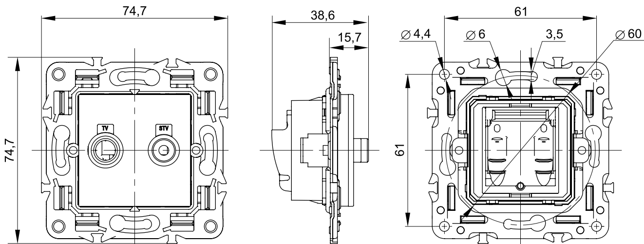
Розетка двухместная TV + SAT
