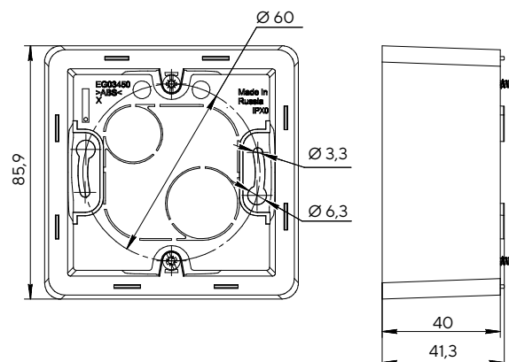
Коробка для накладного монтажа одностенная
