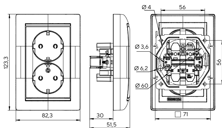
Розетка двухместная с заземлением
