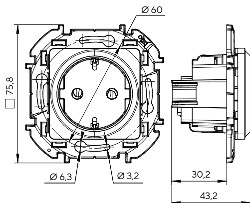
Розетка одноместная с заземлением с защитными шторками
