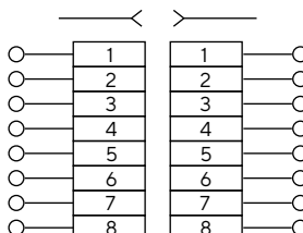
Розетка компьютерная двухместная
