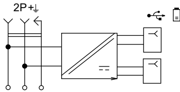
Розетка силовая с USB
