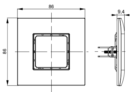
Рамка одноместная
