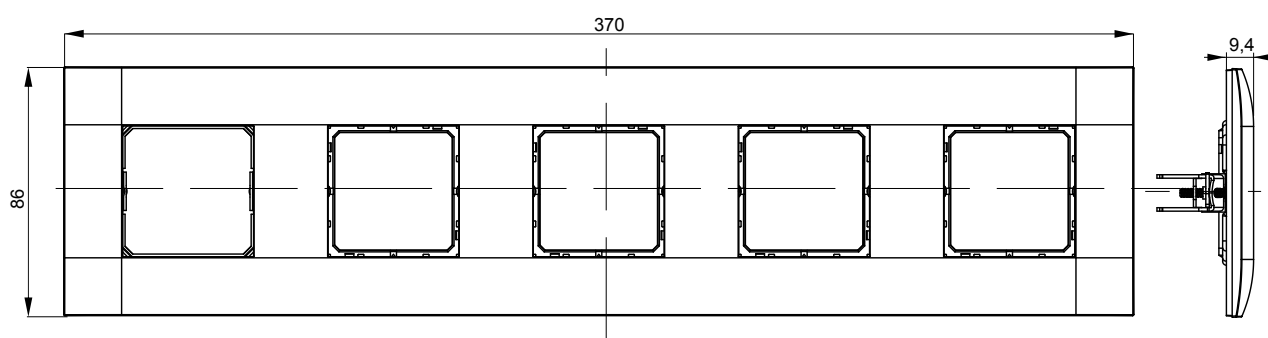
Рамка пятиместная
