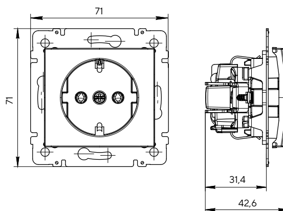
Розетка одностепенная с заземлением
