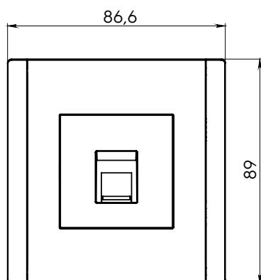
Розетка телефонная RJ11
