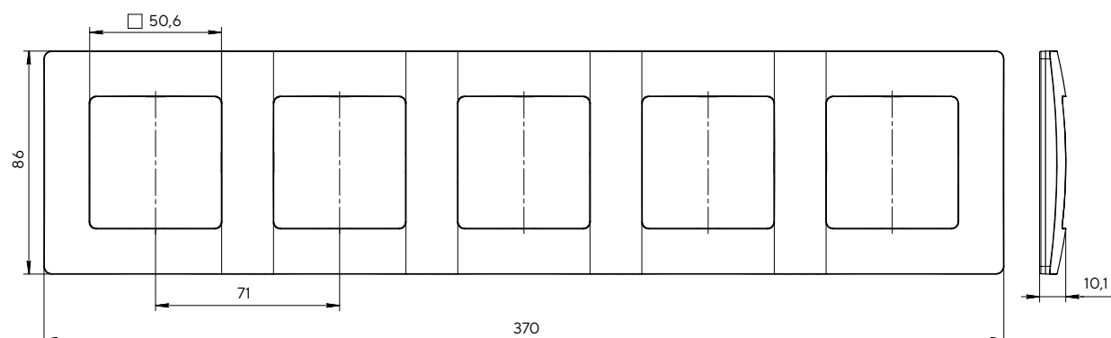
Рамка пятиместная
