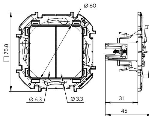
Переключатель двухклавишный
