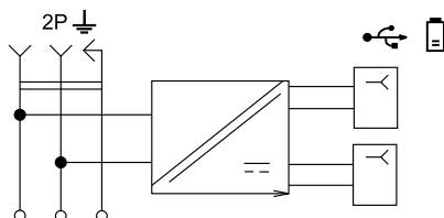
Розетка силовая с USB
