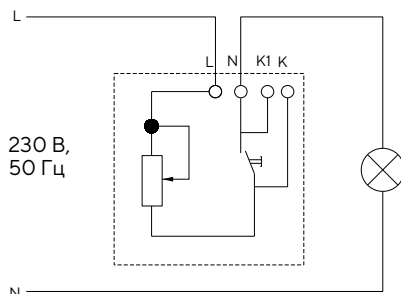
Светорегулятор поворотно-нажимной
