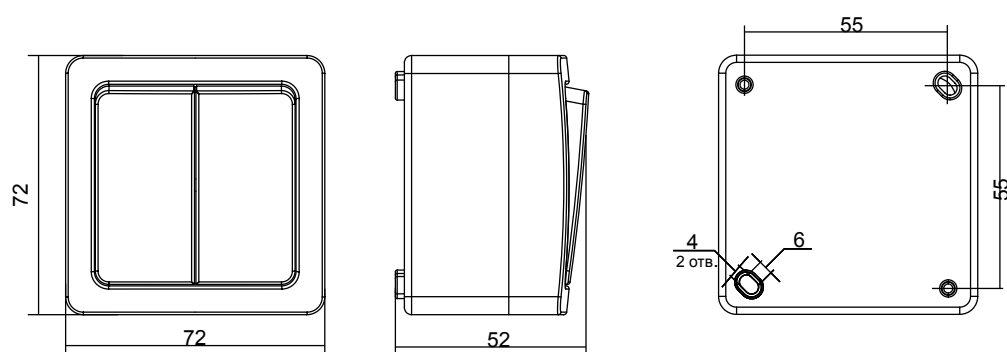
Выключатель двухклавишный
