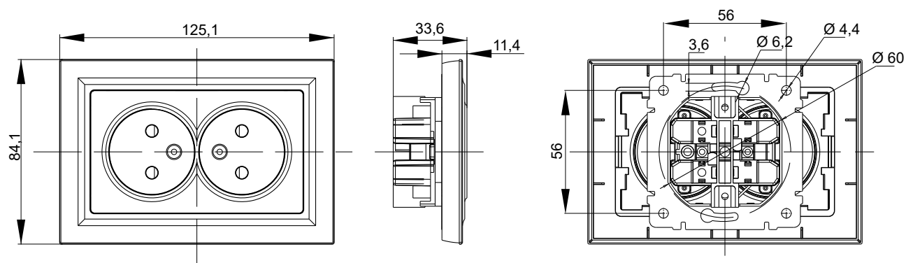
Розетка двухместная без заземления и защитных шторок в сборе
