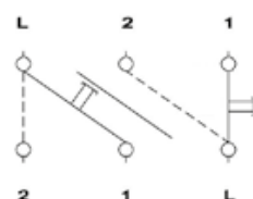
Переключатель двухклавишный самовозвратный
