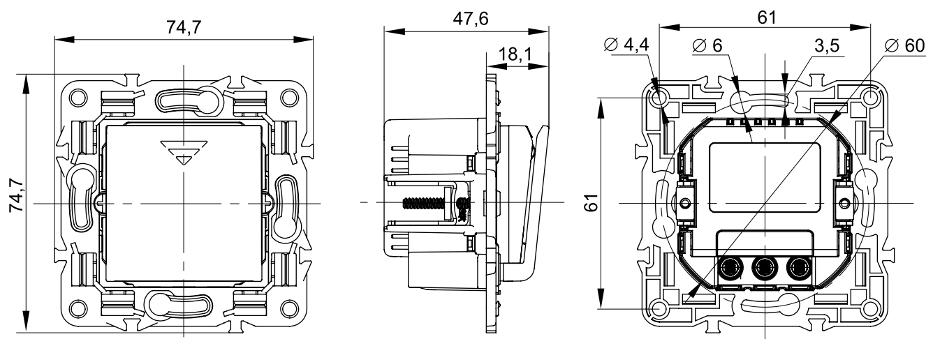
Выключатель карточный
