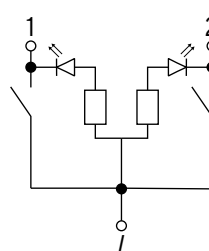
Выключатель двухклавишный с индикацией
