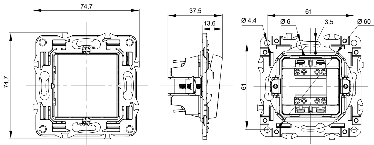
Выключатель одноклавишный
