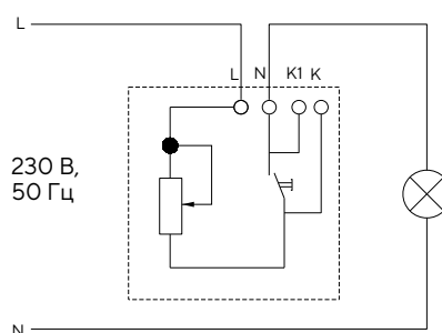
Светорегулятор
