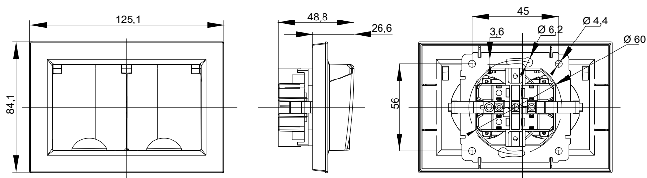
Розетка двухместная с заземлением с защитными шторками и крышкой в сборе
