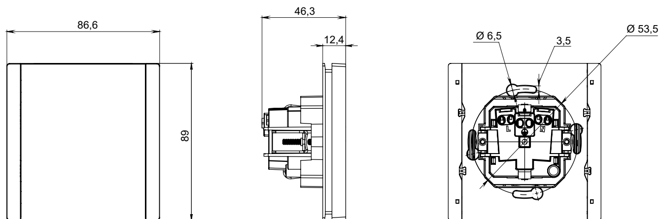
Розетка одностная с крышкой, I_n = 16\text{ A}
