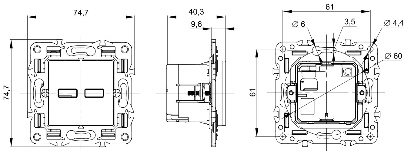
Розетка USB A + A
