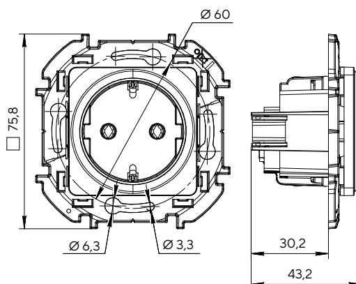
Розетка одноместная с заземлением без защитных шторок
