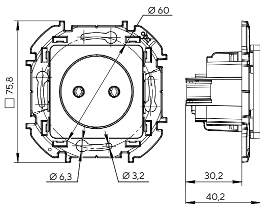
Розетка одноместная без заземления без защитных шторок
