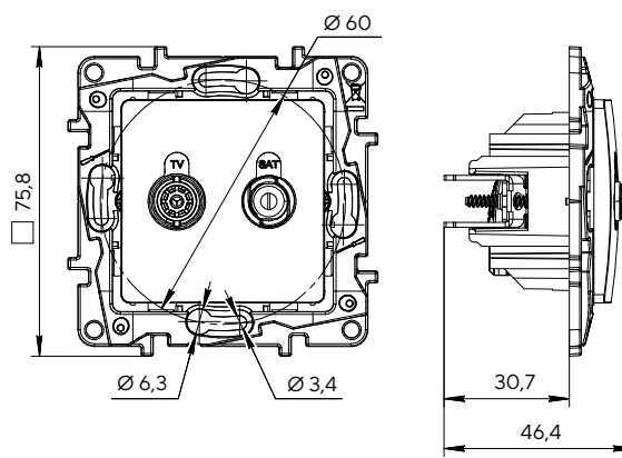
Розетка двухместная TV + SAT
