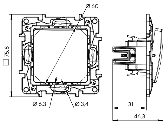
Выключатель одноклавишный
