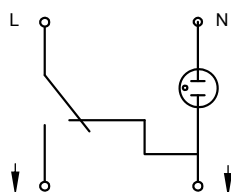
Переключатель одноклавишный с индикацией
