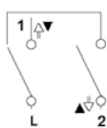
Переключатель для жалюзи с механической блокировкой
