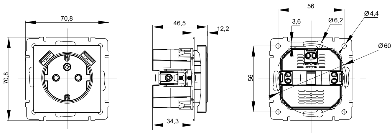
Розетка силовая + 2 USB A + A
