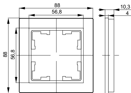
Рамка одноместная
