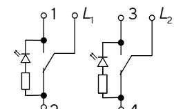
Переключатель двухклавишный проходной с индикацией
