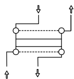
Переключатель одноклавишный перекрестный
