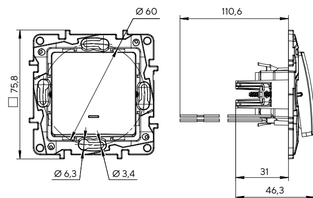
Выключатель одноклавишный с подсветкой/индикацией
