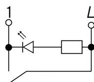
Выключатель одноклавишный с индикацией
