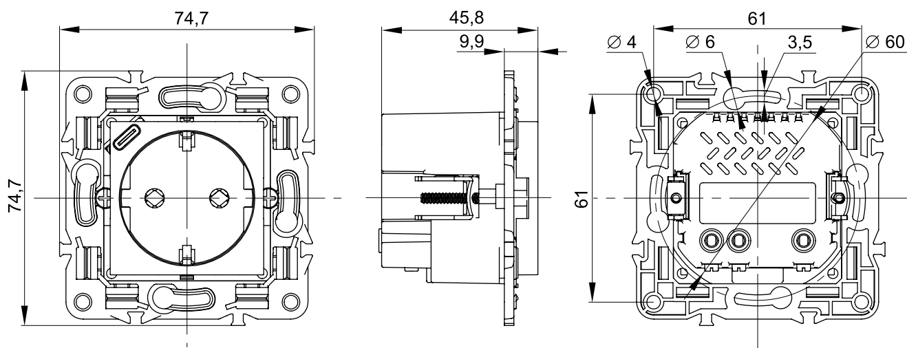
Розетка силовая с заземлением и USB C
