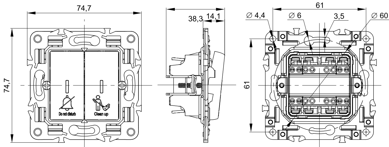
Выключатель двухклавишный с индикацией отельный
