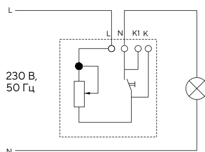
Светорегулятор поворотно-нажимной
