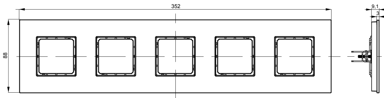
Рамка пятиместная
