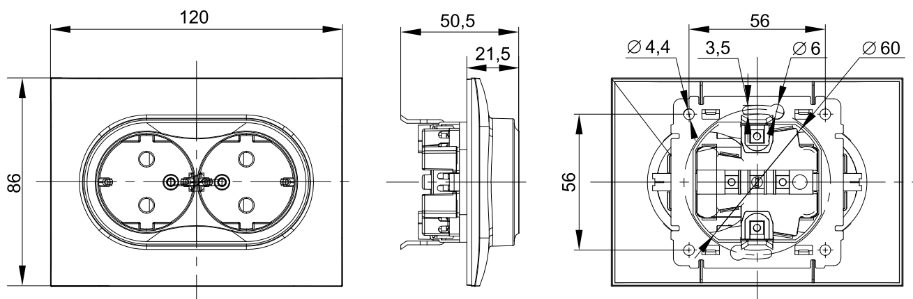
Розетка двухместная с заземлением в пластиковой рамке
