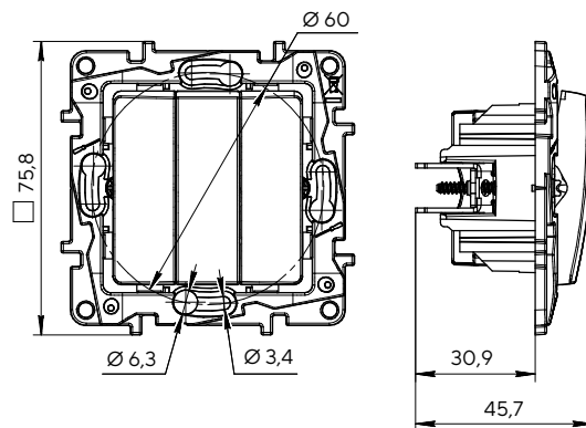
Выключатель трехклавишный
