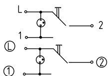
Переключатель двухклавишный кнопочный с индикацией
