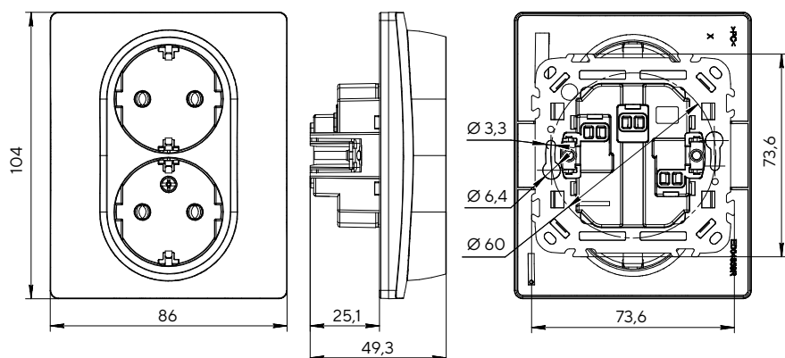
Розетка двухместная с заземлением без защитных шторок в сборе
