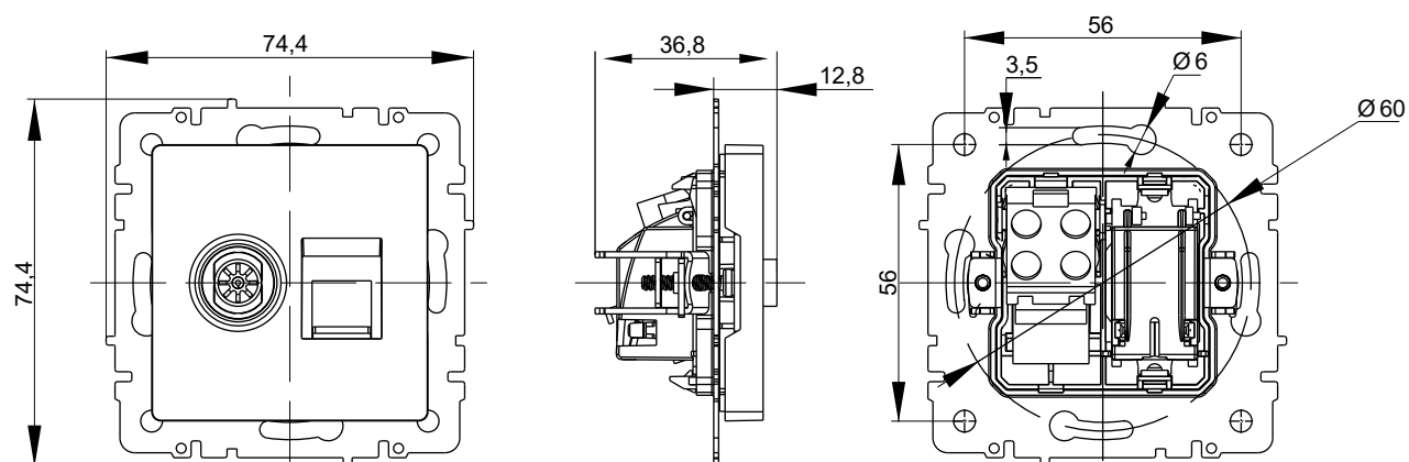
Двухместная (компьютерная + телевизионная) розетка
