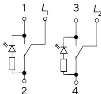
Выключатель двухклавишный с индикацией
