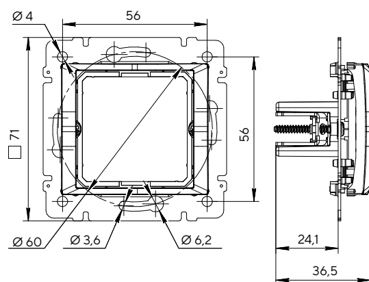
Адаптер для механизмов серии Mosaic
