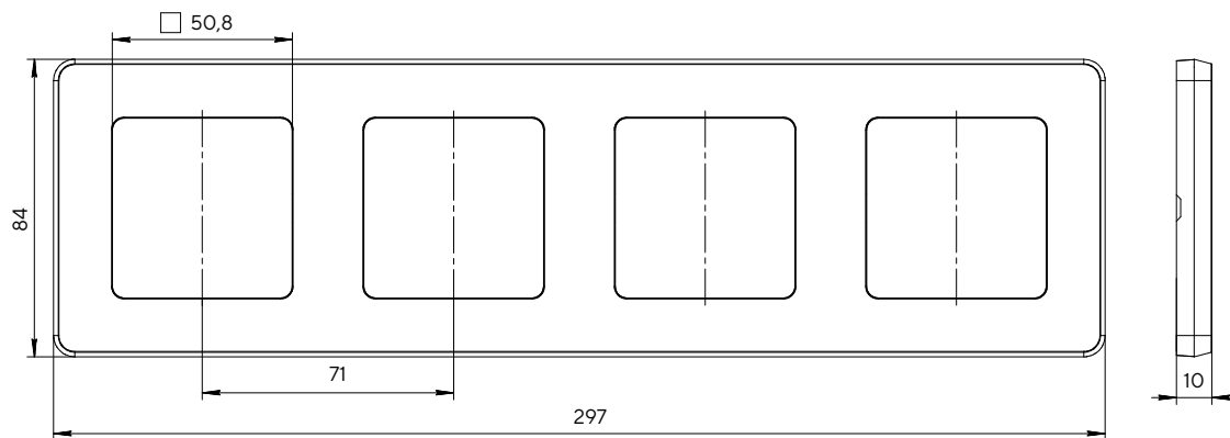
Рамка четырехместная
