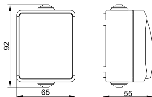
Выключатель одноклавишный
