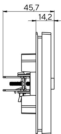
Розетка двухместная TV + компьютерная RJ45
