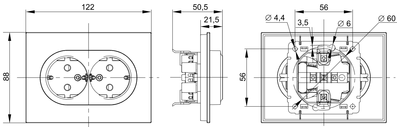
Розетка двухместная с заземлением в стеклянной или металлической рамке
