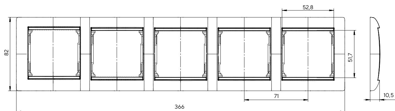
Рамка пятиместная
