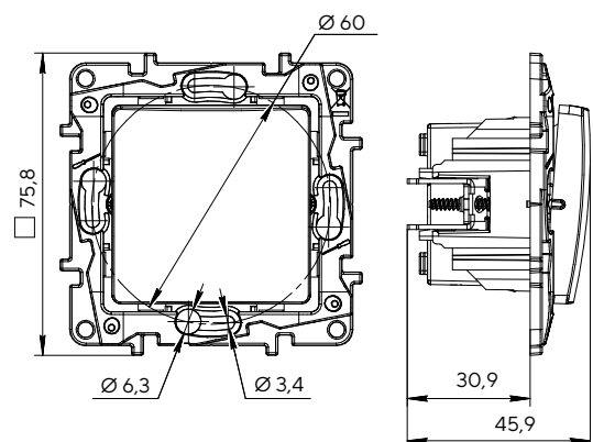
Переключатель одноклавишный перекрестный
