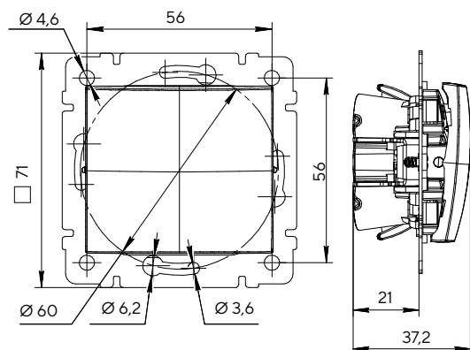
Переключатель одноклавишный, переключатель двухклавишный
