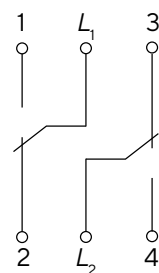
Переключатель двухклавишный
