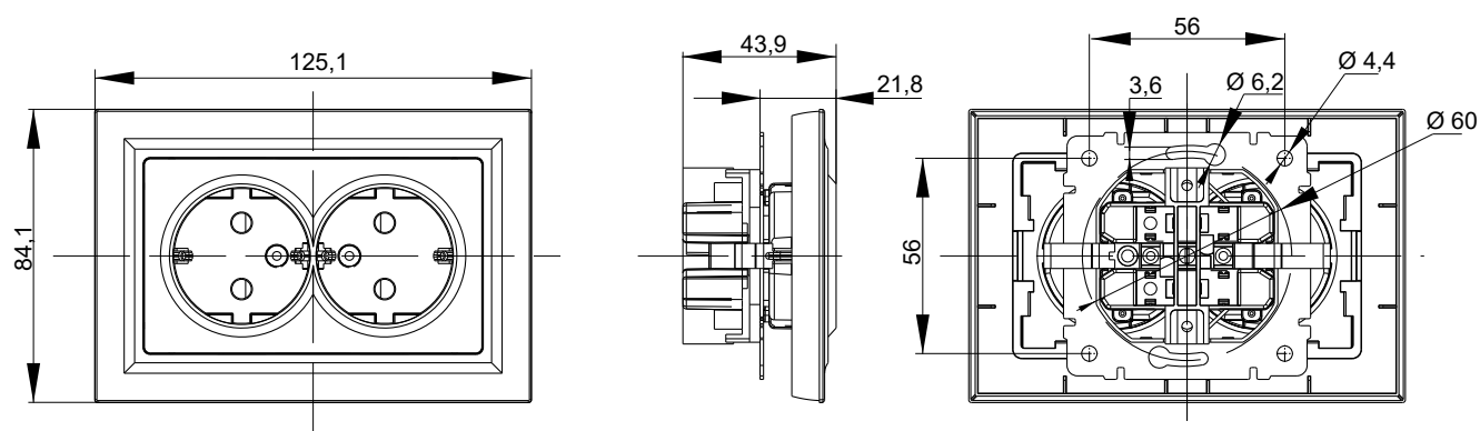
Розетка двухместная с заземлением с защитными шторками в сборе
