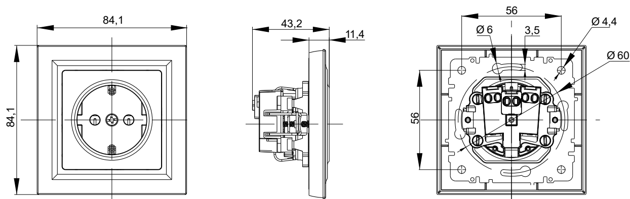
Розетка одноместная с заземлением и защитными шторками в сборе
