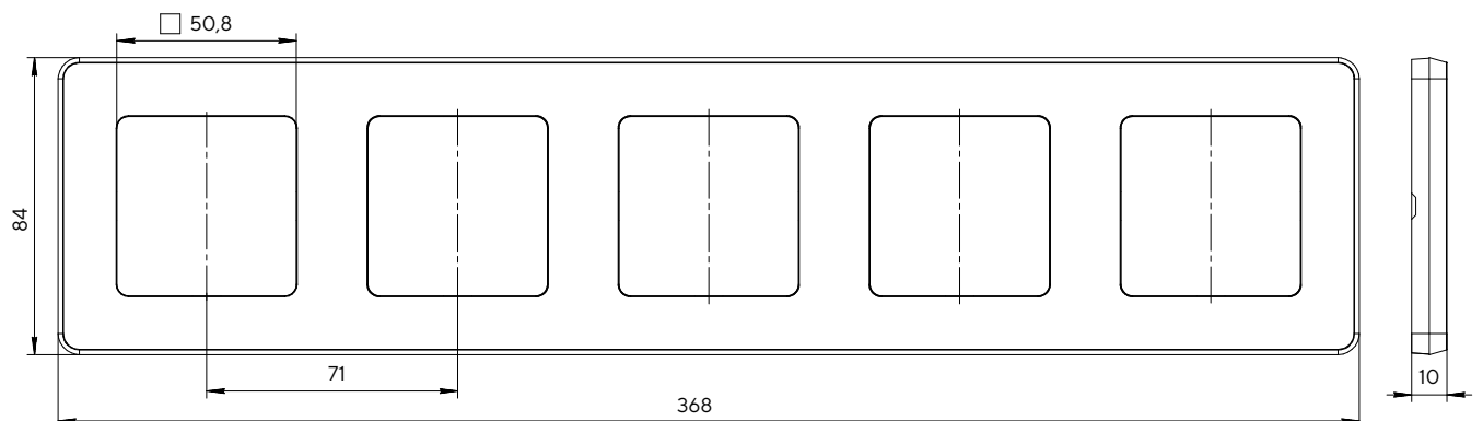
Рамка пятиместная
