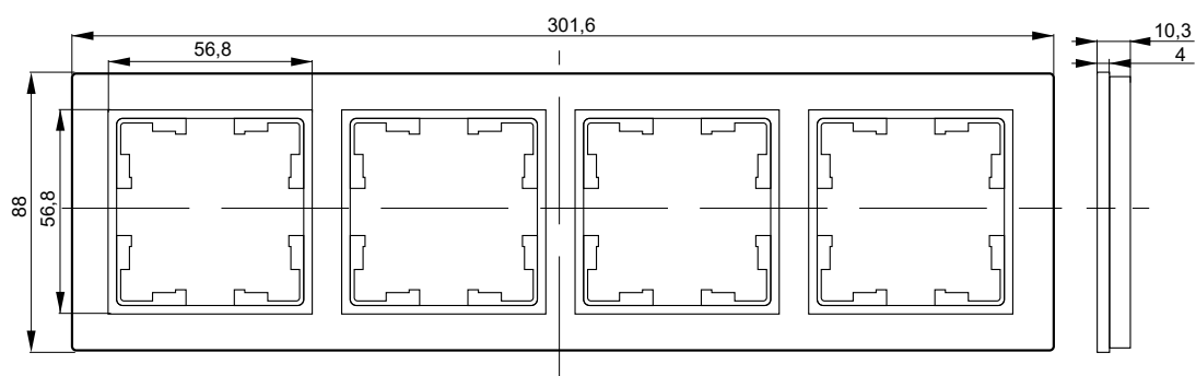
Рамка четырехместная
