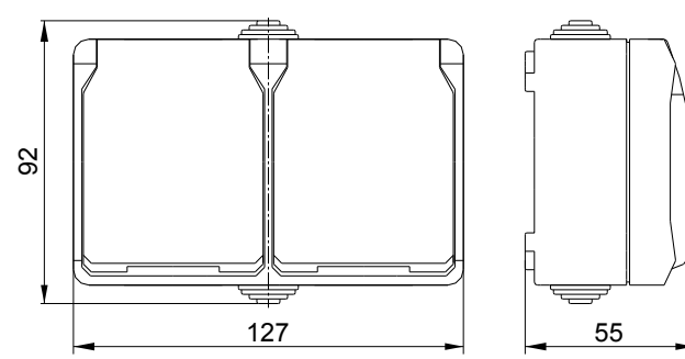
Розетка двухместная
