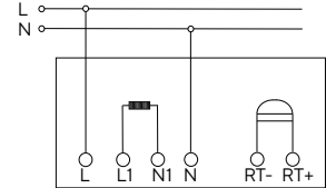
Термостат
