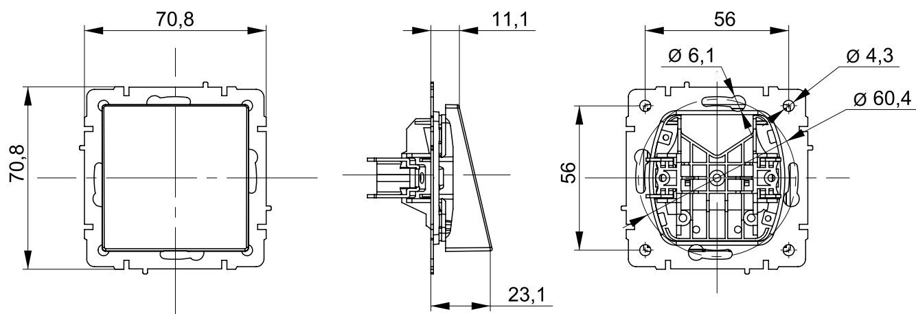
Вывод кабеля встраиваемый
