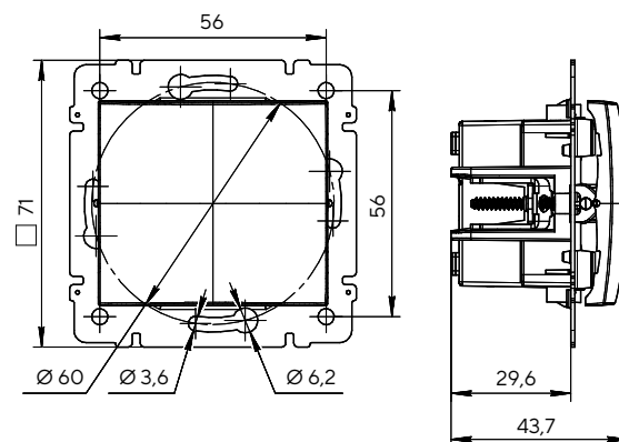
Переключатель перекрестный одноклавишный
