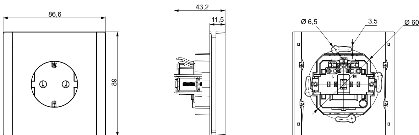
Розетка одностная, безвинтовой зажим, I_n = 16\text{ A}
