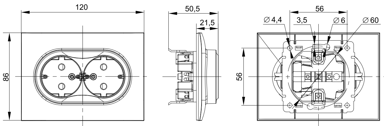
Розетка двухместная с крышкой
