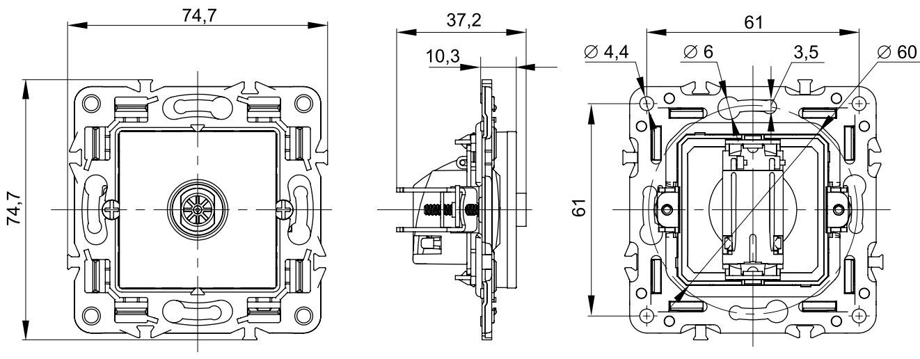
Розетка телевизионная
