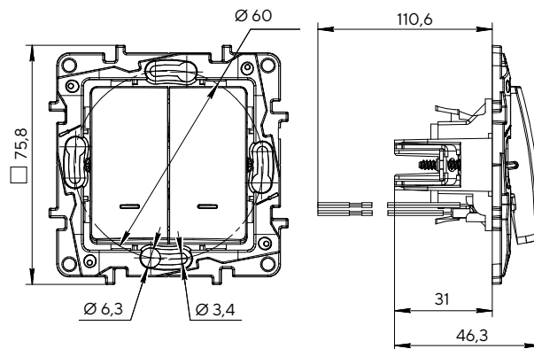
Выключатель двухклавишный с подсветкой/индикацией
