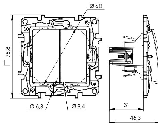
Выключатель двухклавишный
