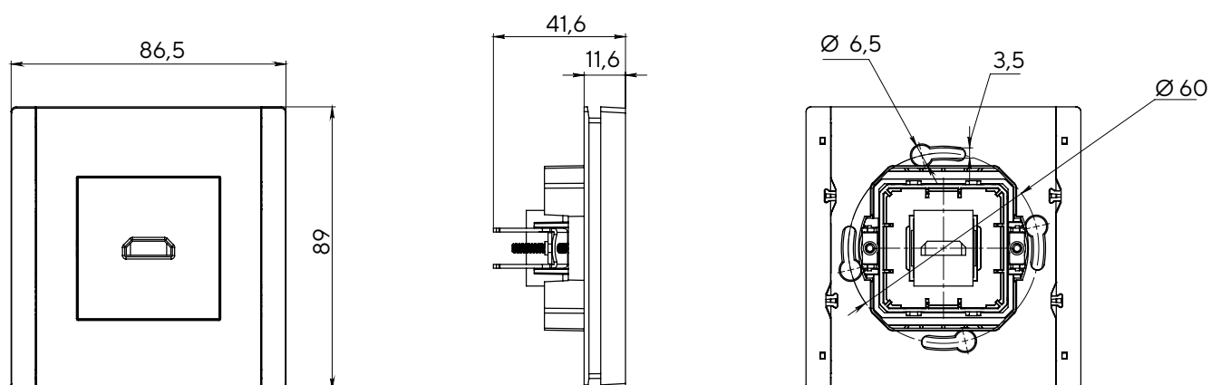
Розетка HDMI
