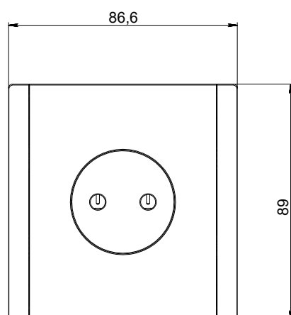
Розетка одноместная, I_n = 10\text{ А}
