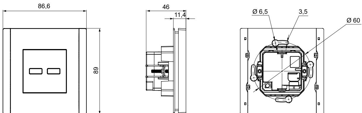
Розетка USB A + C
