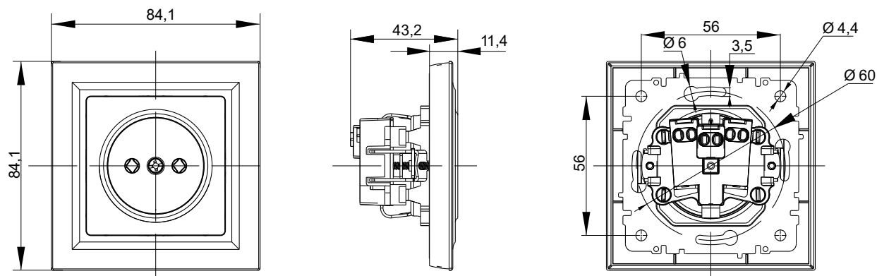
Розетка одноместная без заземления и защитных шторок в сборе
