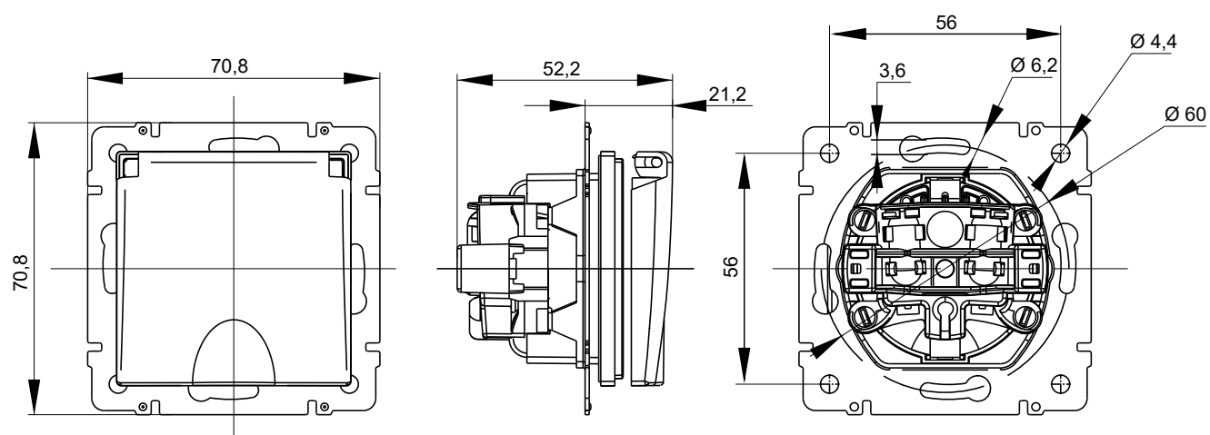
Розетка одноместная с крышкой
