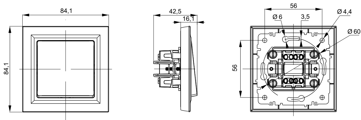
Выключатель в сборе
