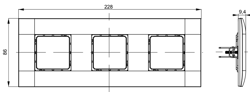
Рамка трехместная
