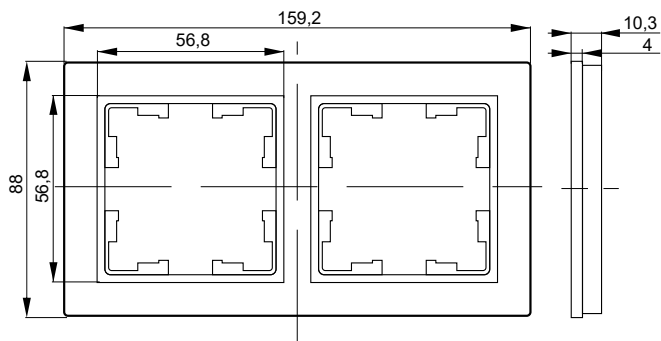
Рамка двухместная
