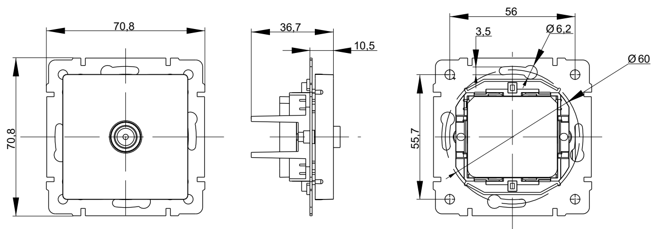
Телевизионная розетка
