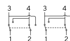
Переключатель двухклавишный перекрестный
