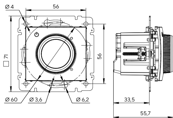
Терморегулятор
