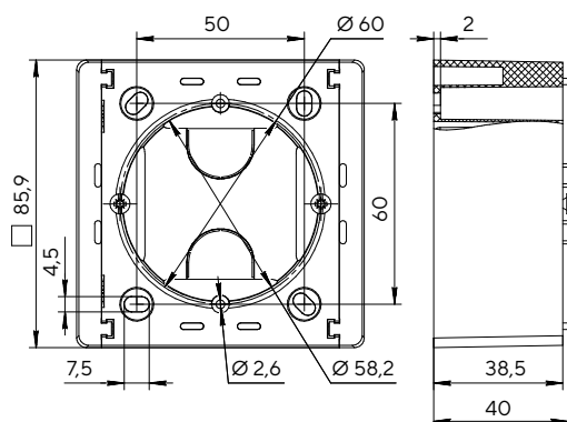
Коробка для накладного монтажа одностная универсальная
