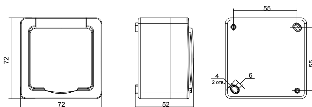
Розетка одноместная
