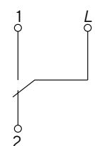
Переключатель одноклавишный проходной
