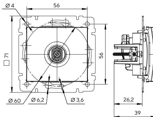
Розетка телевизионная
