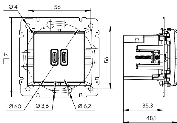
Розетка USB C + C
