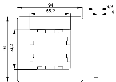
Рамка одноместная
