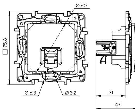
Розетка компьютерная RJ45
