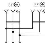
Розетка двухместная с заземлением
