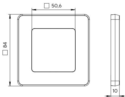
Рамка одноместная
