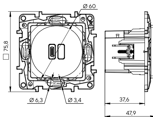
Розетка USB C
