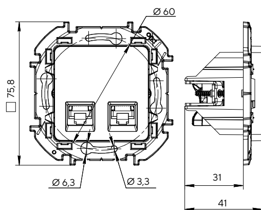
Розетка компьютерная двухместная RJ45
