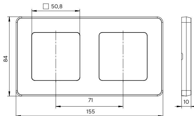
Рамка двухместная
