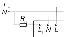
Терморегулятор
