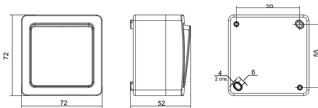
Выключатель одноклавишный
