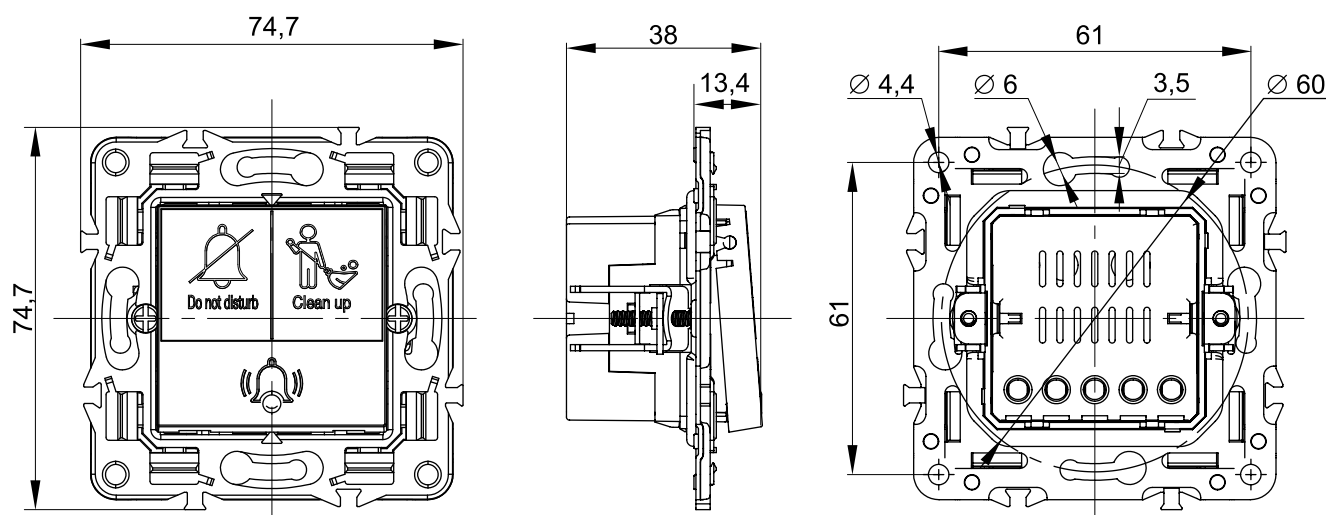
Кнопка вызова персонала с индикацией отельная
