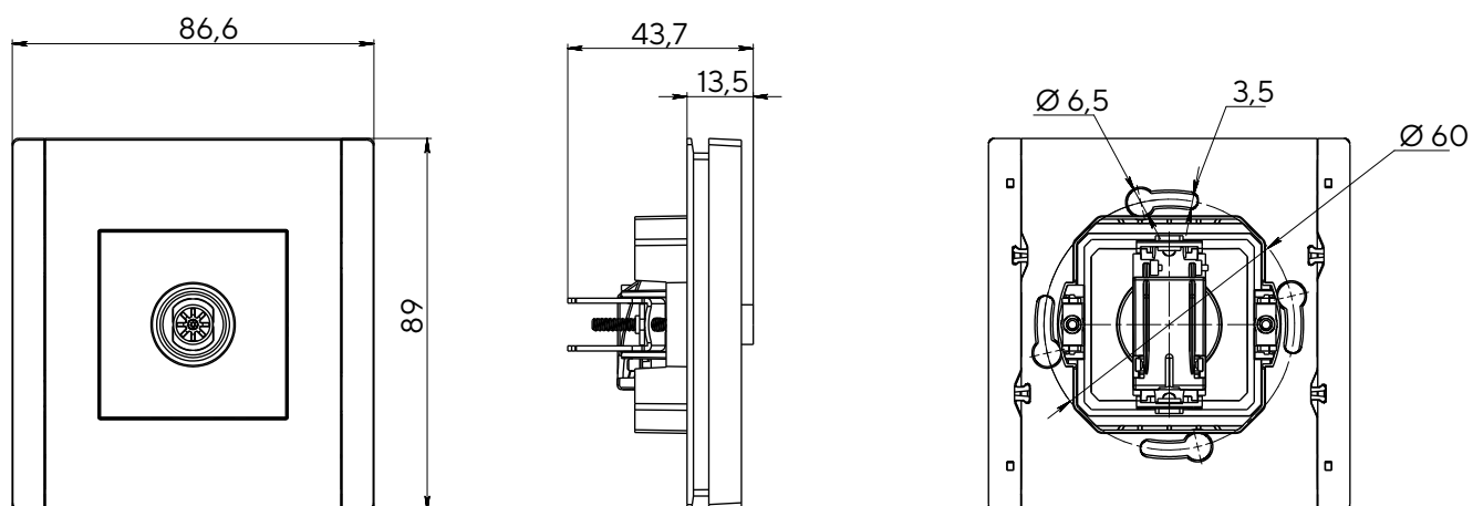
Розетка телевизионная
