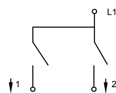
Выключатель двухклавишный
