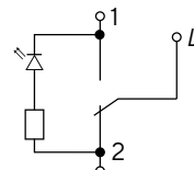
Выключатель самовозвратный
