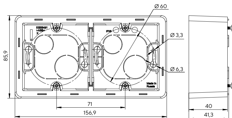
Коробка для накладного монтажа двухстенная
