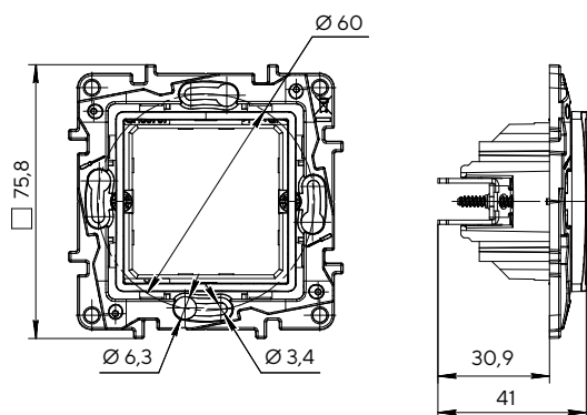
Адаптер для механизмов серии Mosaic
