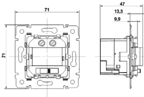
Датчик движения
