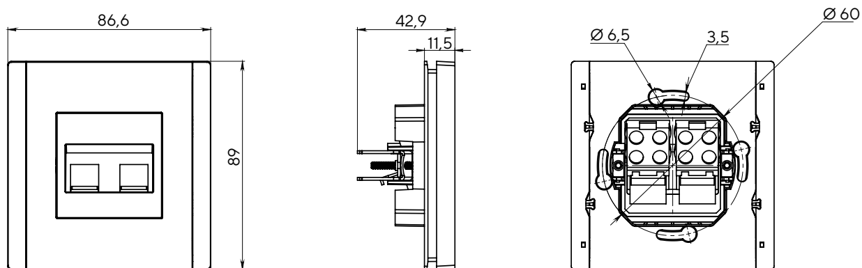
Розетка USB A + A
