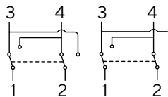
Переключатель двухклавишный проходной
