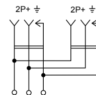
Розетка двухместная
