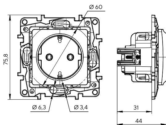
Розетка одноместная с заземлением без защитных шторок
