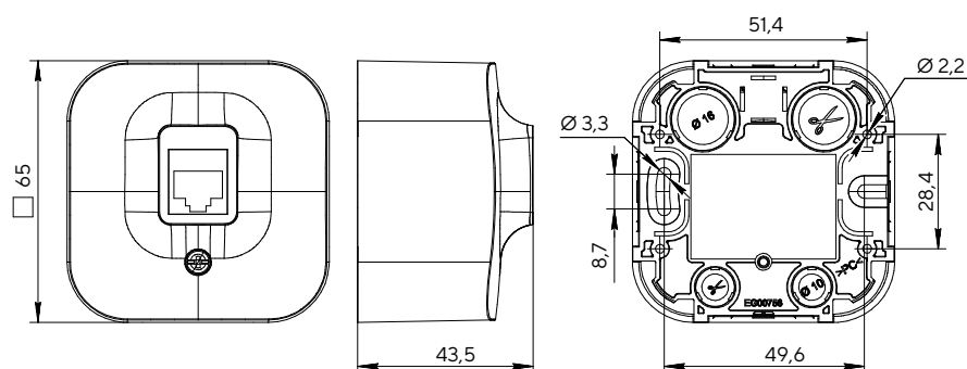
Розетка компьютерная/телефонная RJ45
