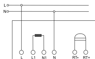
Термостат
