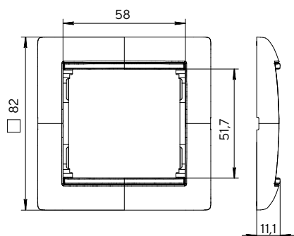
Рамка одноместная
