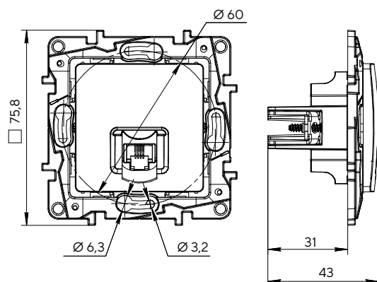
Розетка телефонная RJ11
