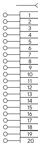
Розетка HDMI
