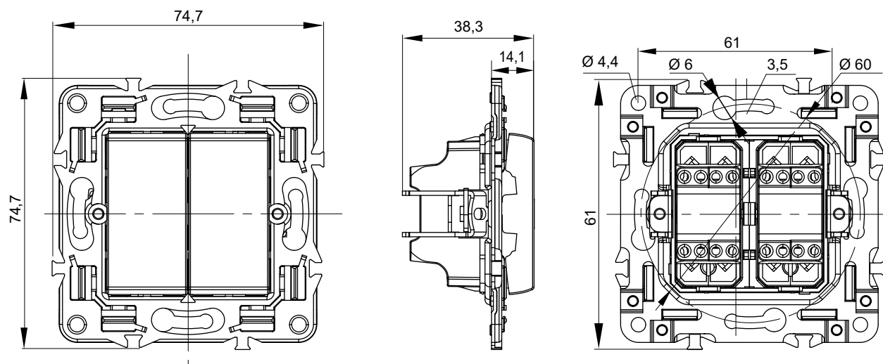
Выключатель двухклавишный
