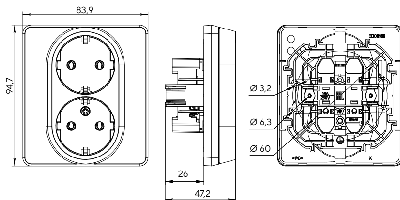
Розетка двухместная с заземлением без защитных шторок в сборе
