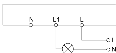
Датчик движения
