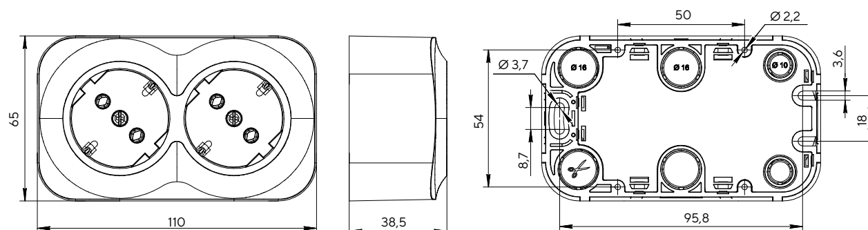
Розетка двухместная с заземлением без защитных шторок
