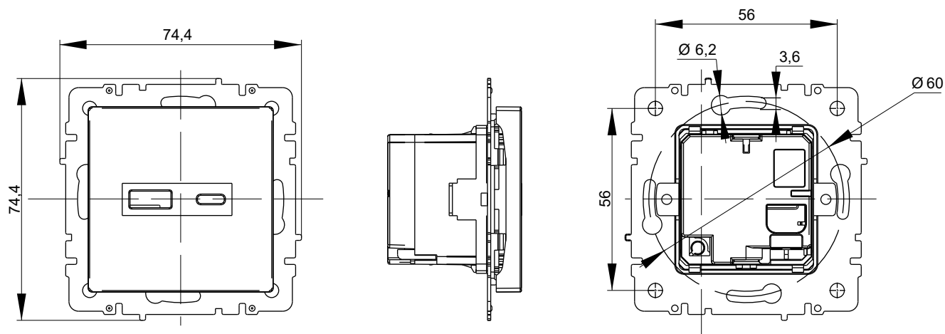
Розетка USB A + C
