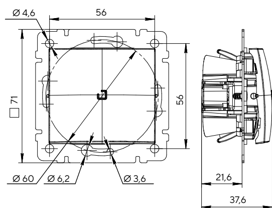
Выключатель/переключатель самовозвратный для жалюзи двухклавишный
