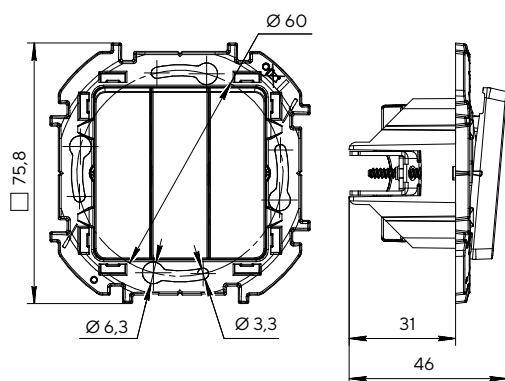
Выключатель трехклавишный
