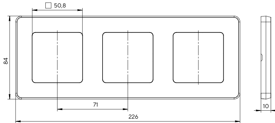
Рамка трехместная
