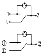
Переключатель двухклавишный с индикацией
