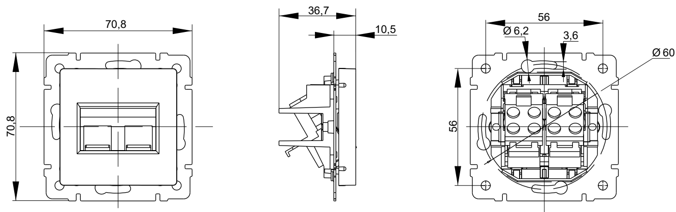
Двухместная (компьютерная + телефонная) розетка
