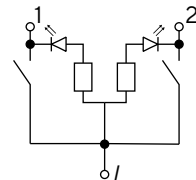
Выключатель двухклавишный с индикацией
