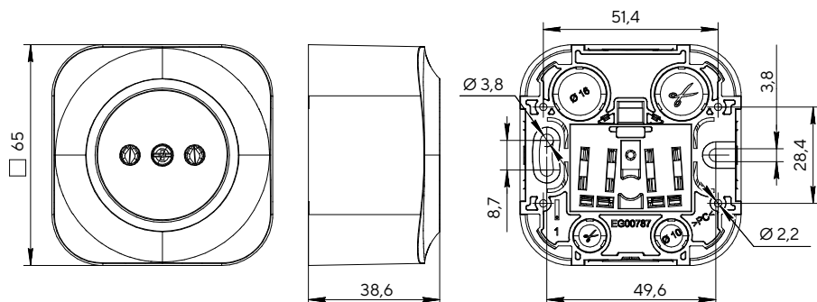
Розетка одностная без заземления без защитных шторок
