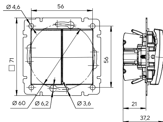
Выключатель/переключатель самовозвратный для жалюзи двухклавишный
