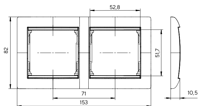
Рамка двухместная
