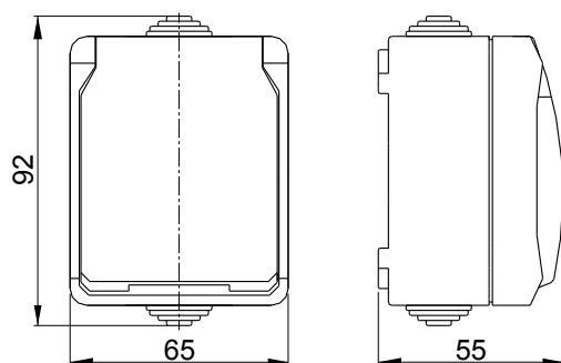
Розетка одноместная
