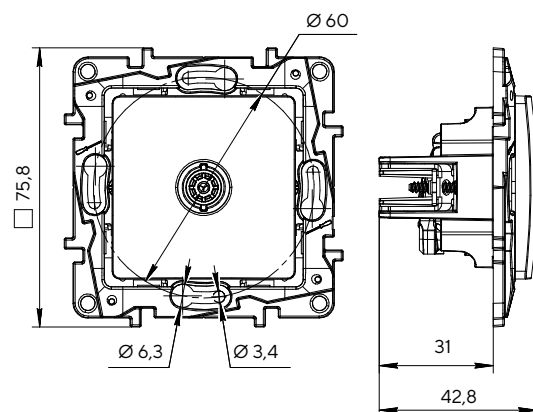
Розетка телевизионная
