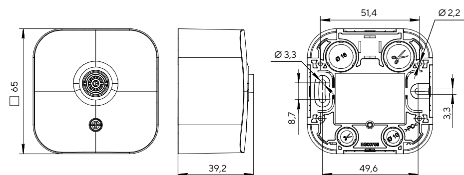
Розетка телевизионная
