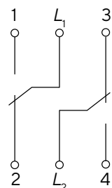
Переключатель двухклавишный проходной
