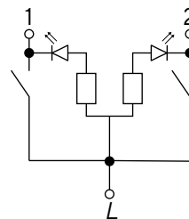
Выключатель двухклавишный с подсветкой/ индикацией
