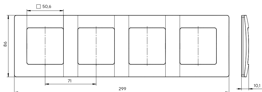
Рамка четырехместная
