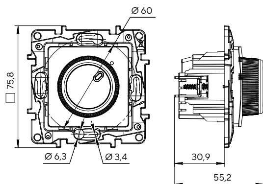
Светорегулятор поворотно-нажимной
