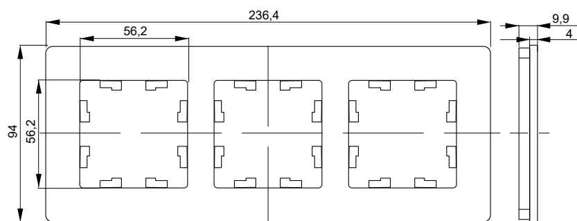
Рамка 3 поста
