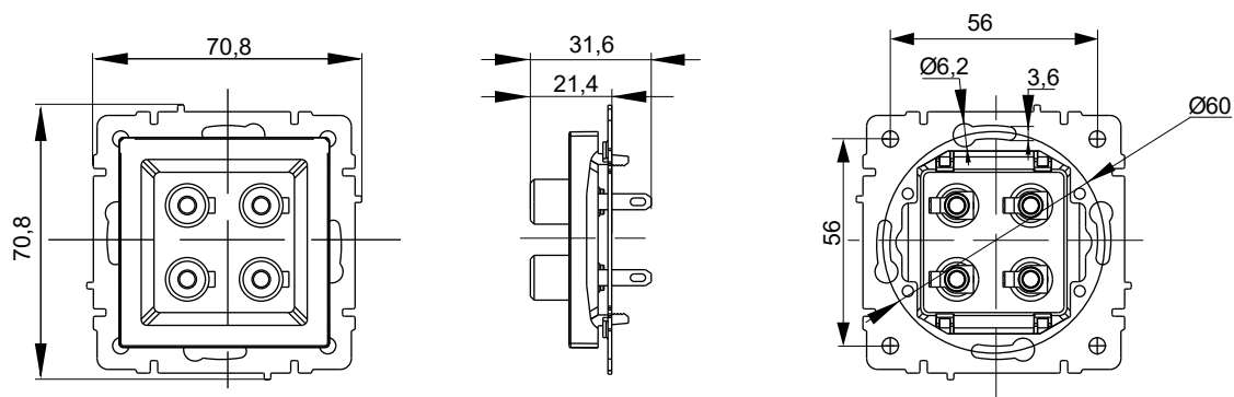
Розетка акустическая
