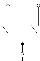
Выключатель двухклавишный
