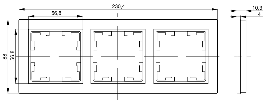
Рамка 3 поста
