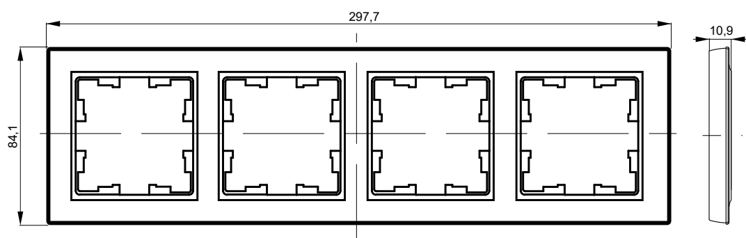
Рамка 4 поста
