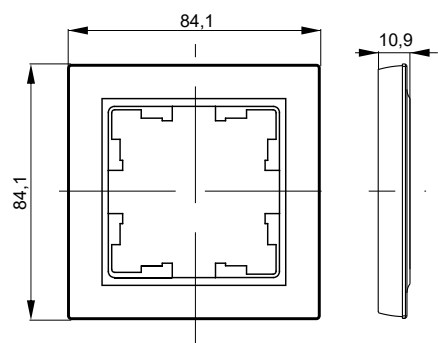
Рамка 1 пост
