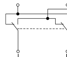
Переключатель одноклавишный
