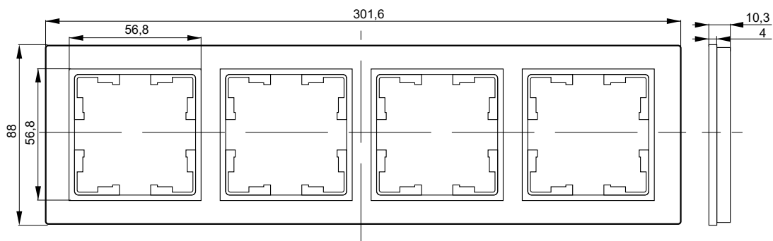
Рамка 4 поста
