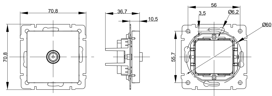
Телевизионная розетка
