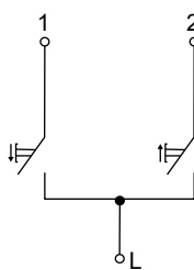
Выключатель жалюзи
