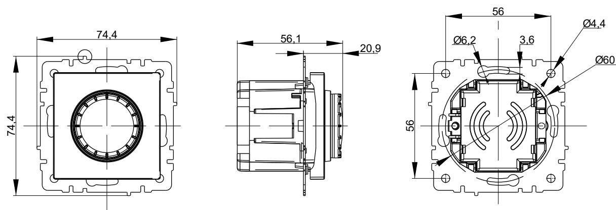
Светорегулятор поворотного-нажимной
