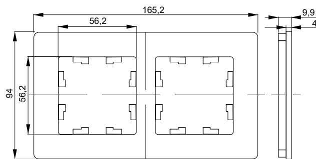
Рамка 2 поста
