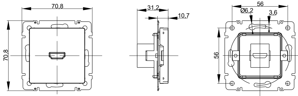
Розетка HDMI
