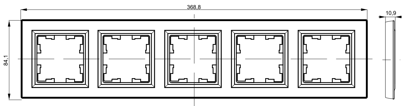
Рамка 5 постов
