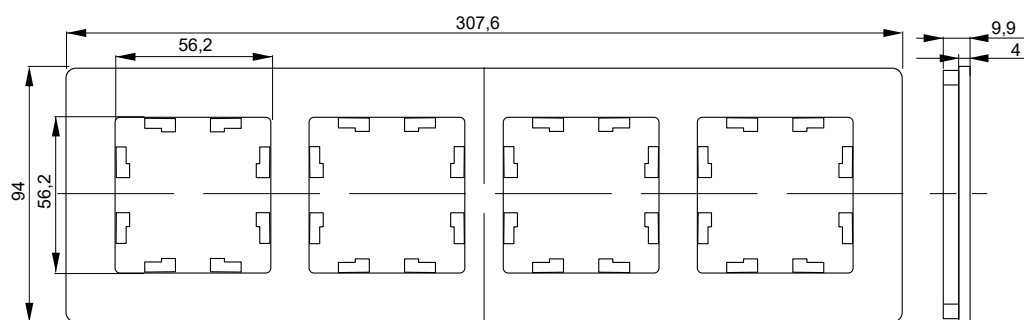
Рамка 4 поста
