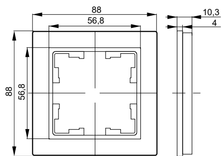
Рамка 1 пост
