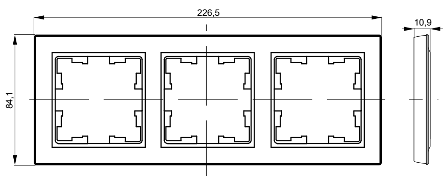
Рамка 3 поста
