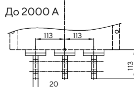
Вид Б (вертикальные выводы)
