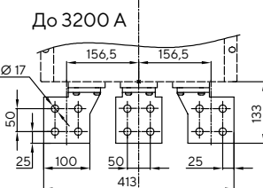
Вид А (горизонтальные выводы)
