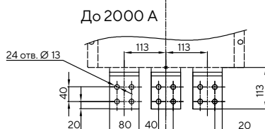
Вид А (горизонтальные выводы)
