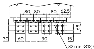
Вид Б (вертикальные выводы)
