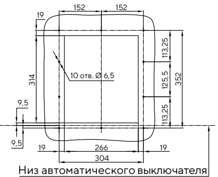
Расположение крепежных отверстий (вид снизу)
