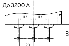
Вид Б (вертикальные выводы)
