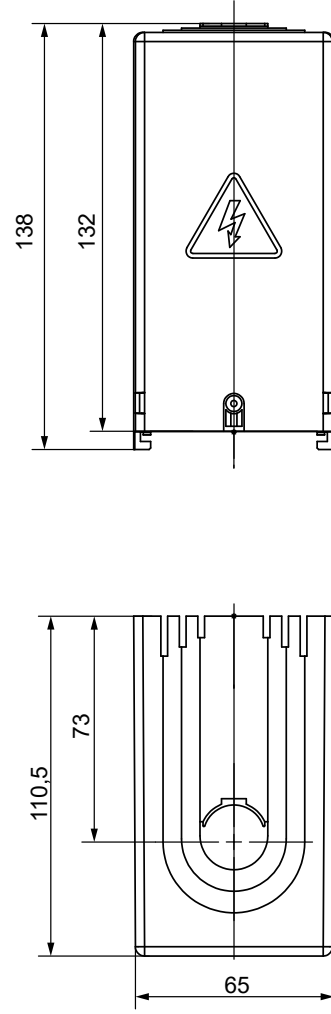
Крышка выводов высокая 630–800 А
