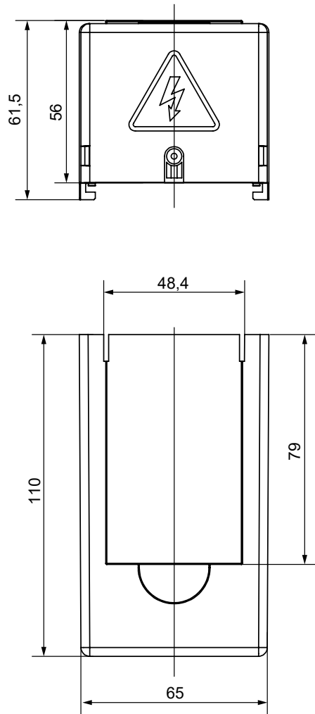
Крышка выводов низкая 630–800 А
