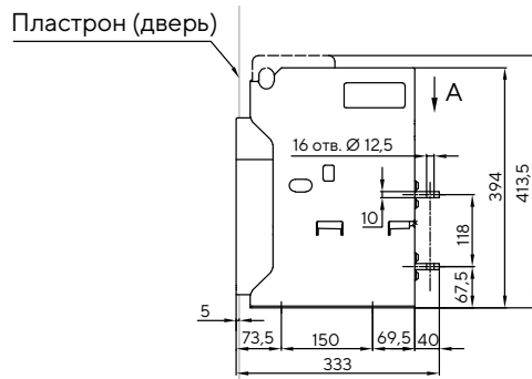
Вид сбоку Вариант 1. Горизонтальные выводы (стандарт)
