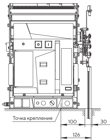
Стационарный автоматический выключатель
