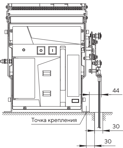
Стационарный автоматический выключатель
