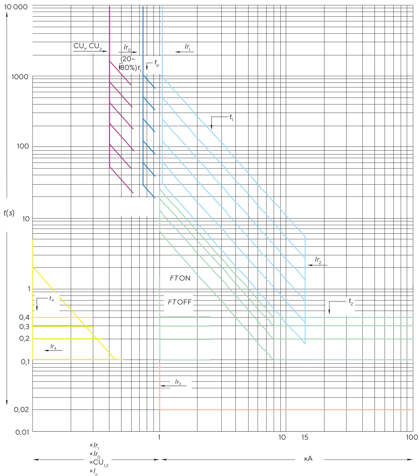
Рисунок 1. Времятоковая характеристика, тип защиты – Pt
