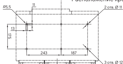
Расположение крепежных отверстий (вид снизу)
