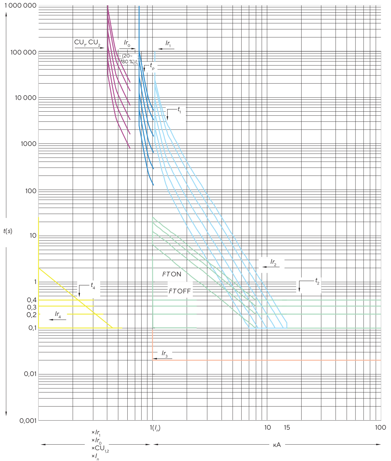
Рисунок 3. Времятоковая характеристика, тип защиты – I^2t^*
