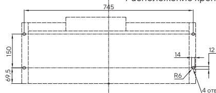
Расположение крепежных отверстий (вид снизу)
