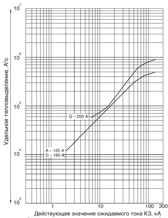
МССВ габаритов А – 125 А, D – 160 А
