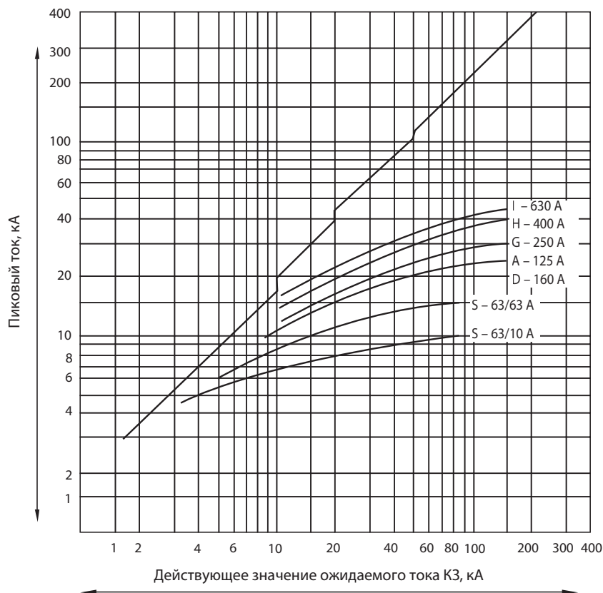
АС 400 В ARMAT МССВ, кривая ограничения тока КЗ, кА (удар.)
