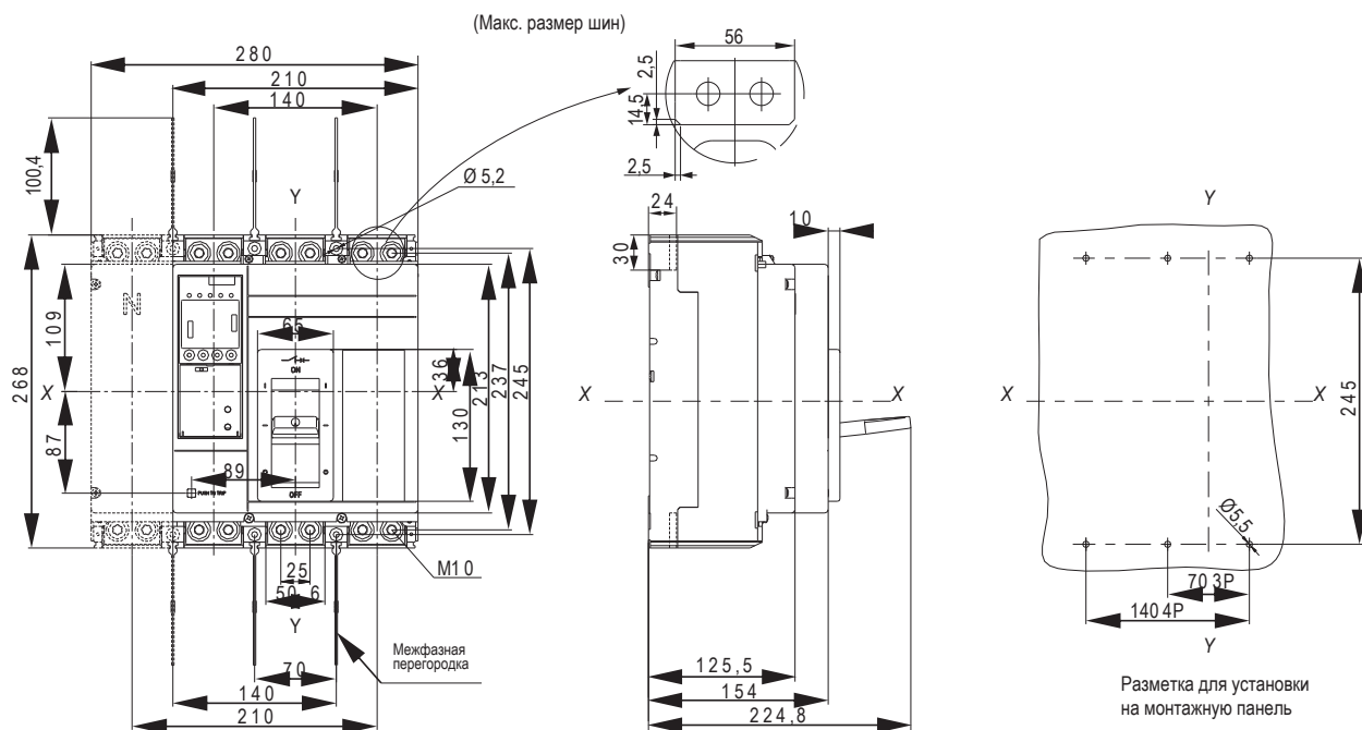
МССВ типоразмера N
