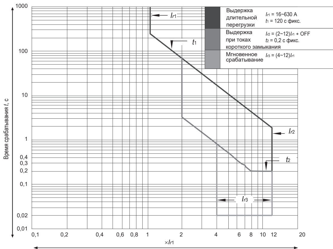
МССВ типоразмеров А, D, G, Н, I с электронным расцепителем ELSC
