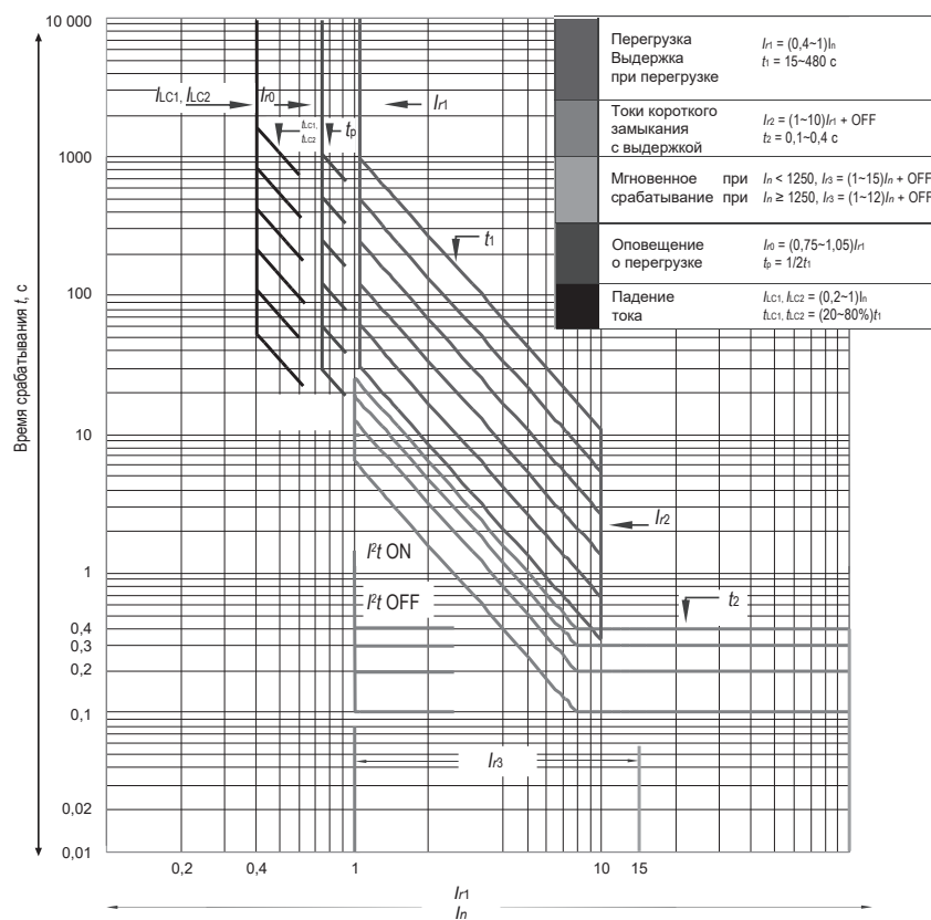
МССВ типоразмера N с электронными расцепителями ELSC, ELPC
