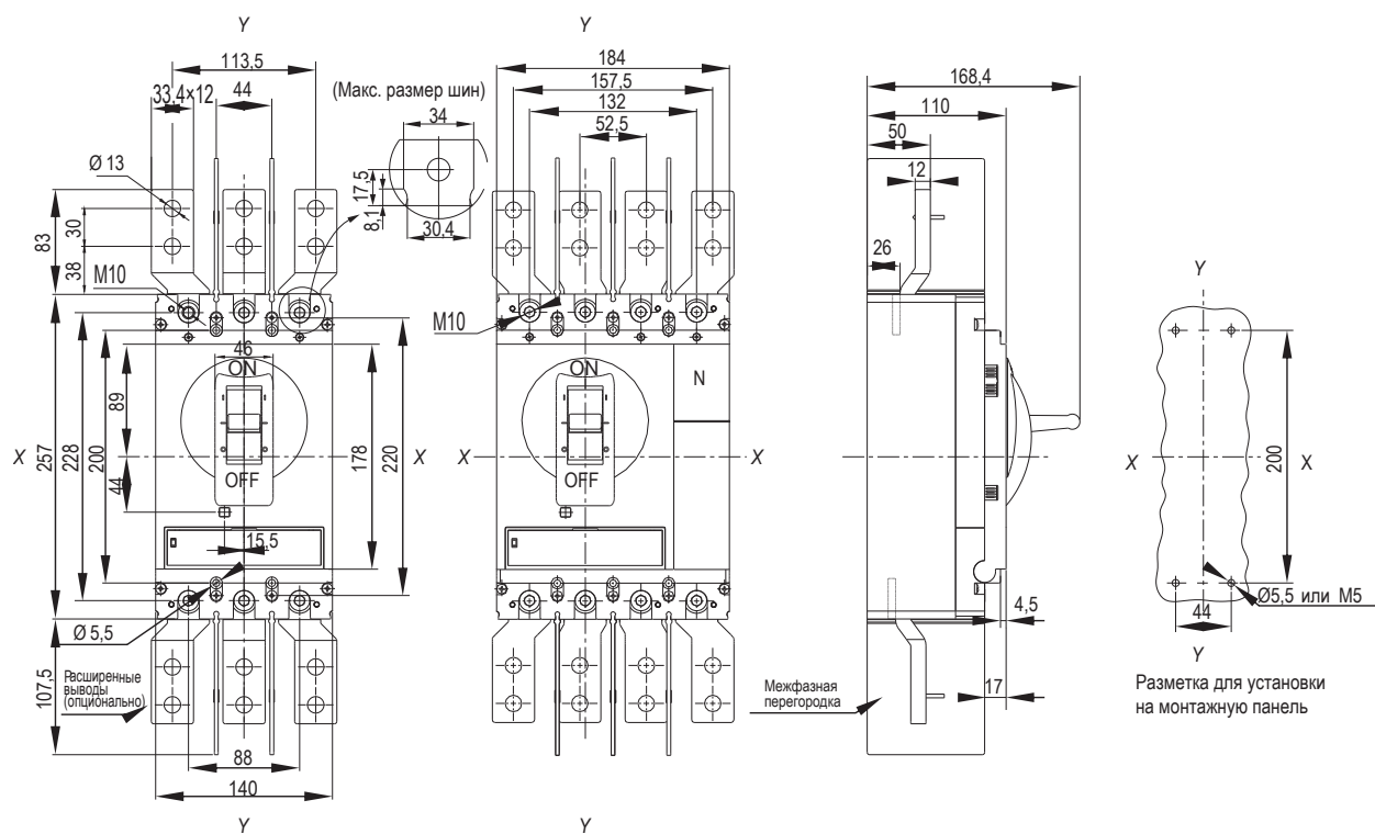
МССВ типоразмера H и I
