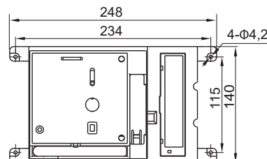
Электропривод типоразмеров H, I
