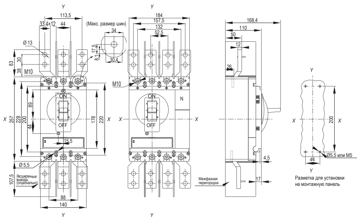
МССВ типоразмера Н, I
