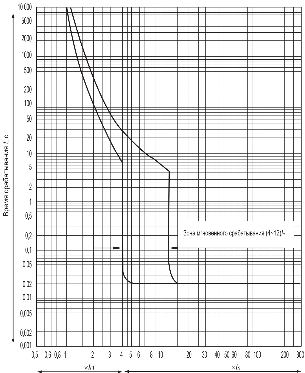
Времятоковые характеристики МССВ типоразмера D ( I_{nm} = 160\text{ A} )
