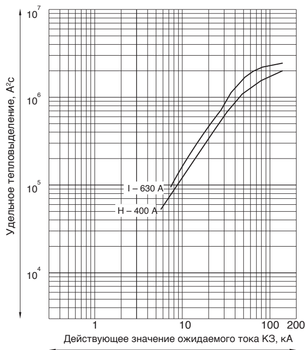
МССВ габаритов H – 400 А, I – 630 А
