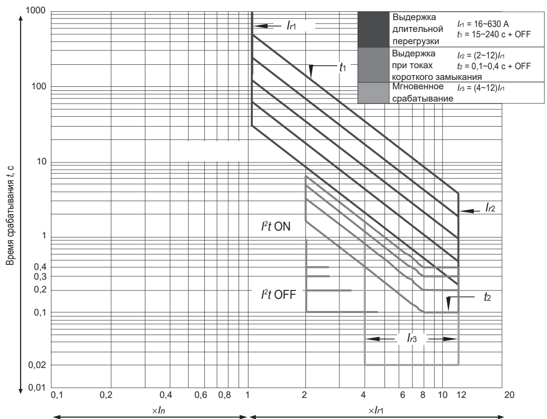
МССВ типоразмеров А, D, G, Н, I с электронным расцепителем ELPC
