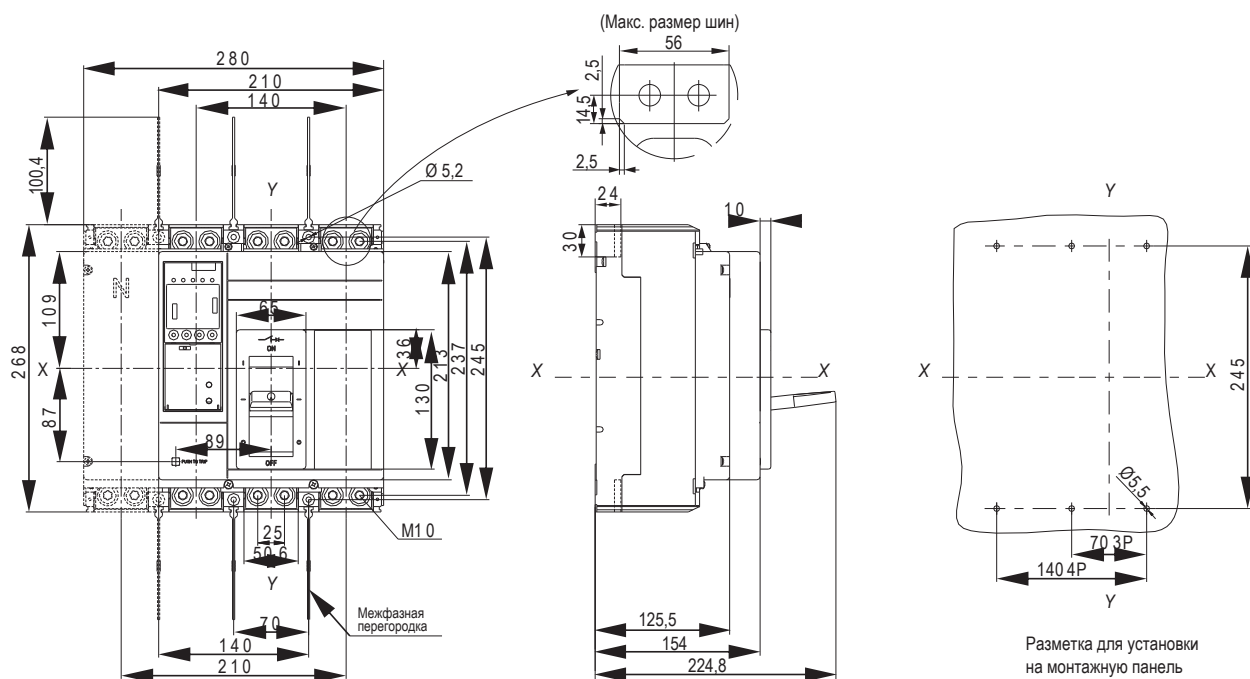
МССВ типоразмера N
