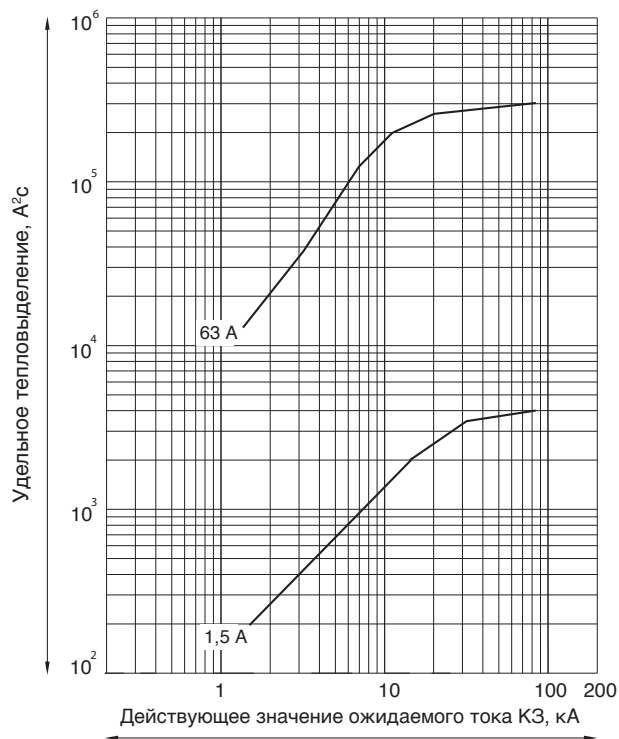
МССВ габарита S, 63 А
