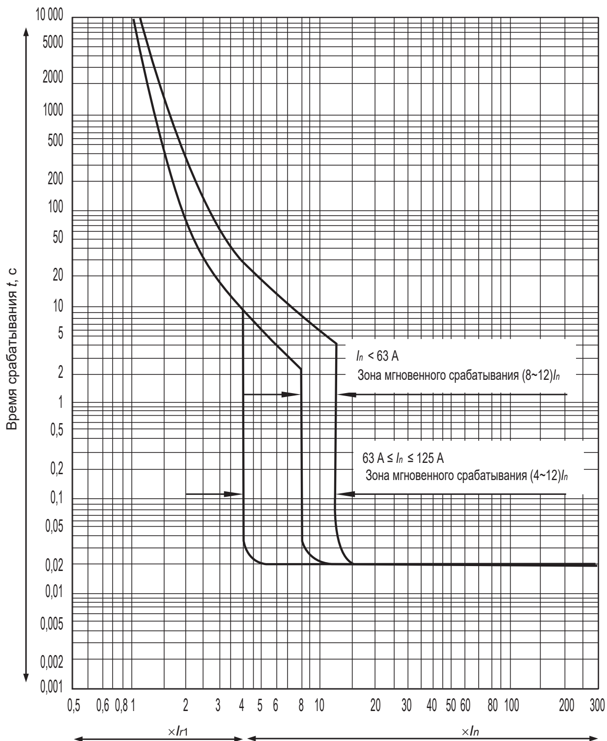
Времятоковые характеристики МССВ типоразмера А ( I_{nm} = 125\text{ A} )
