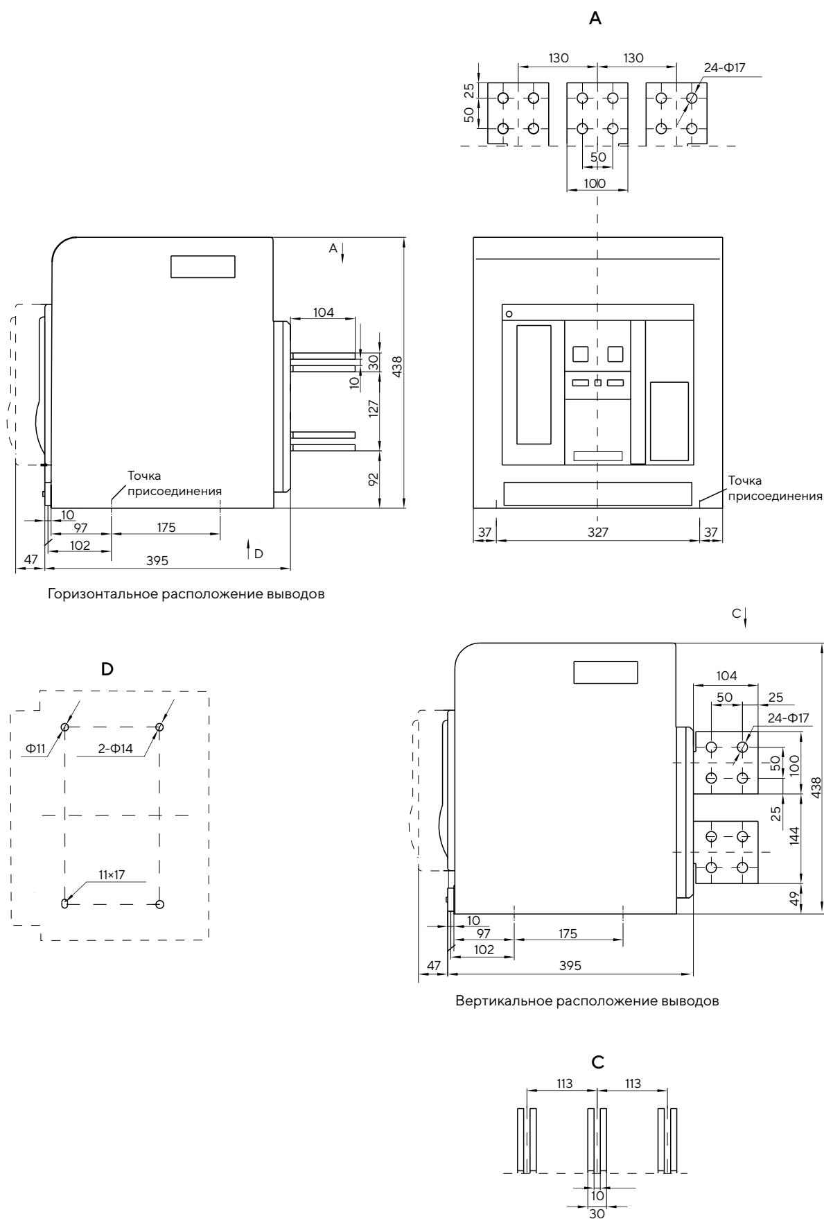
Рис. В.8. Габаритные размеры выдвижных трехполюсных выключателей типоразмера Е (2500~3200 А)
