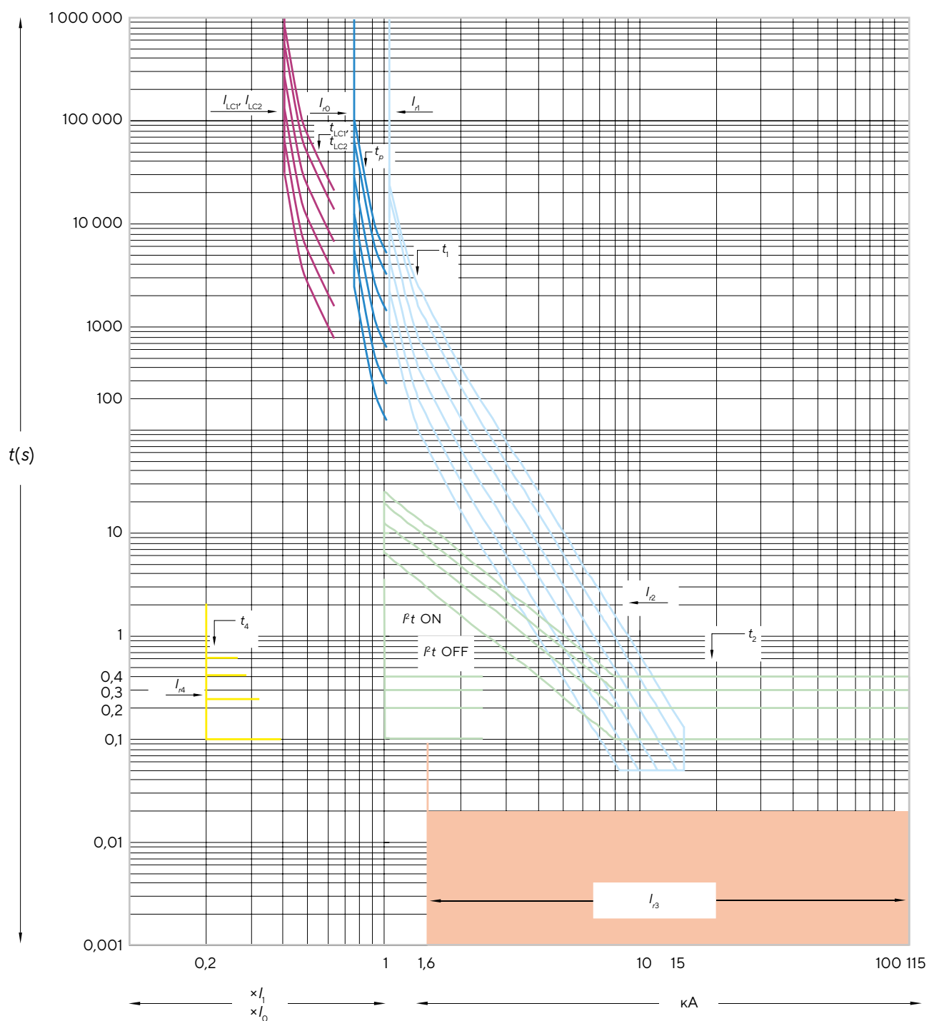
Рис. А.3. Времятоковая характеристика, тип защиты - I^2t
