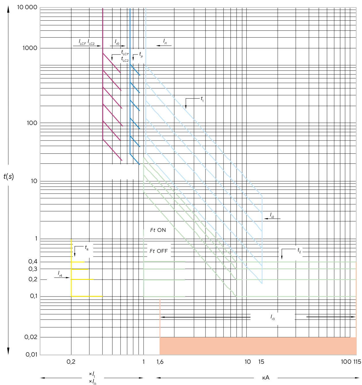
Рис. А.1. Времятоковая характеристика, тип защиты - I^2t
