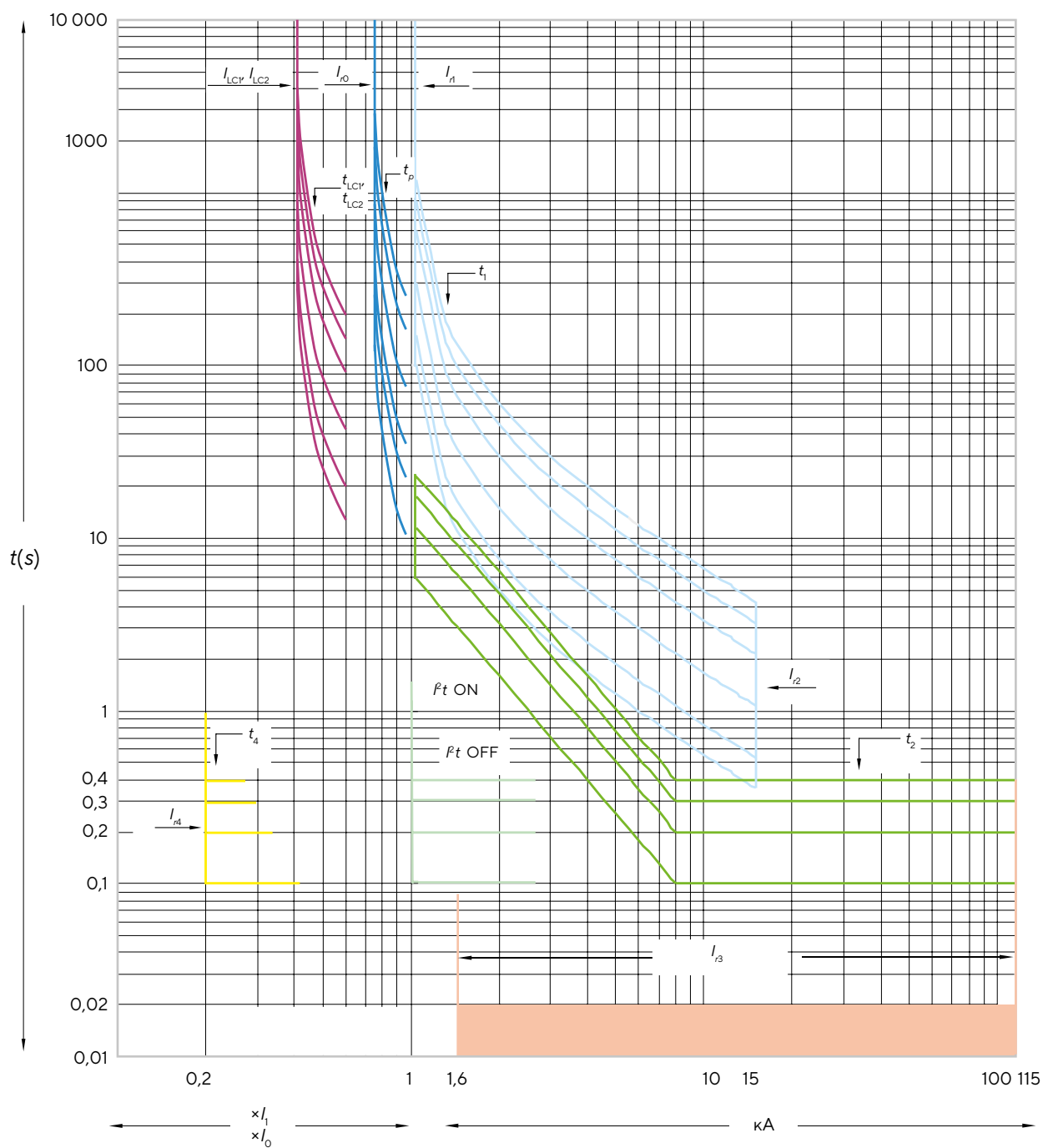
Рис. А.2. Времятоковая характеристика, тип защиты - I t
