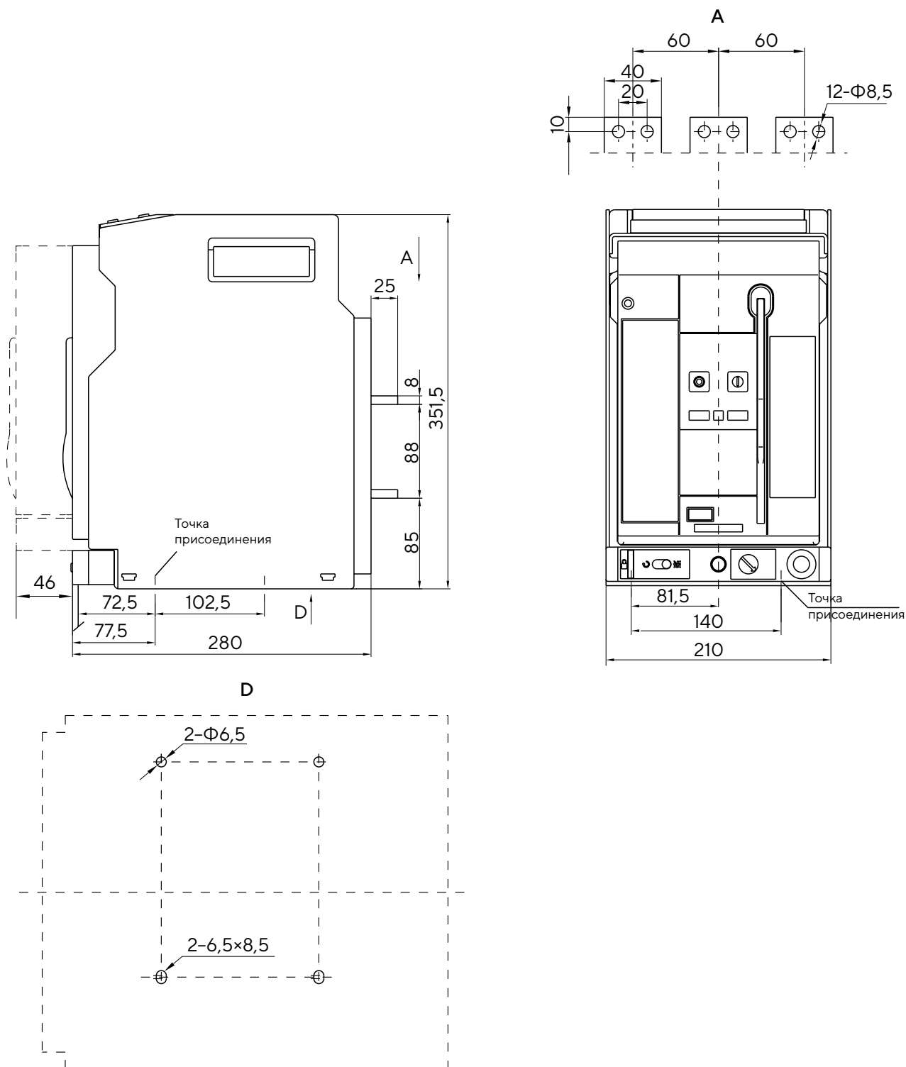
Рис. В.1. Габаритные размеры выдвижных трехполюсных выключателей типоразмера S
