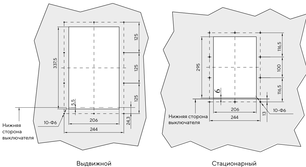
Рис. В.13. Габаритные размеры рамки обрамления выреза в двери для выключателей типоразмера S
