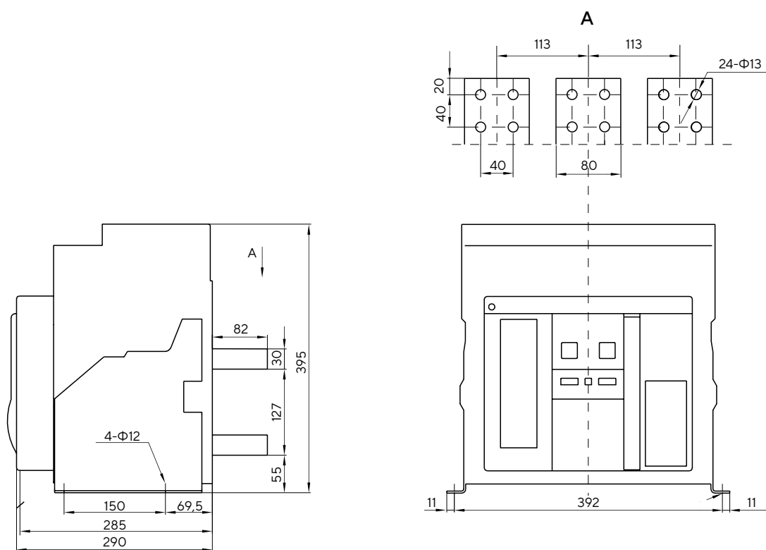
Рис. В.12. Габаритные размеры стационарных трехполюсных выключателей типоразмера F
