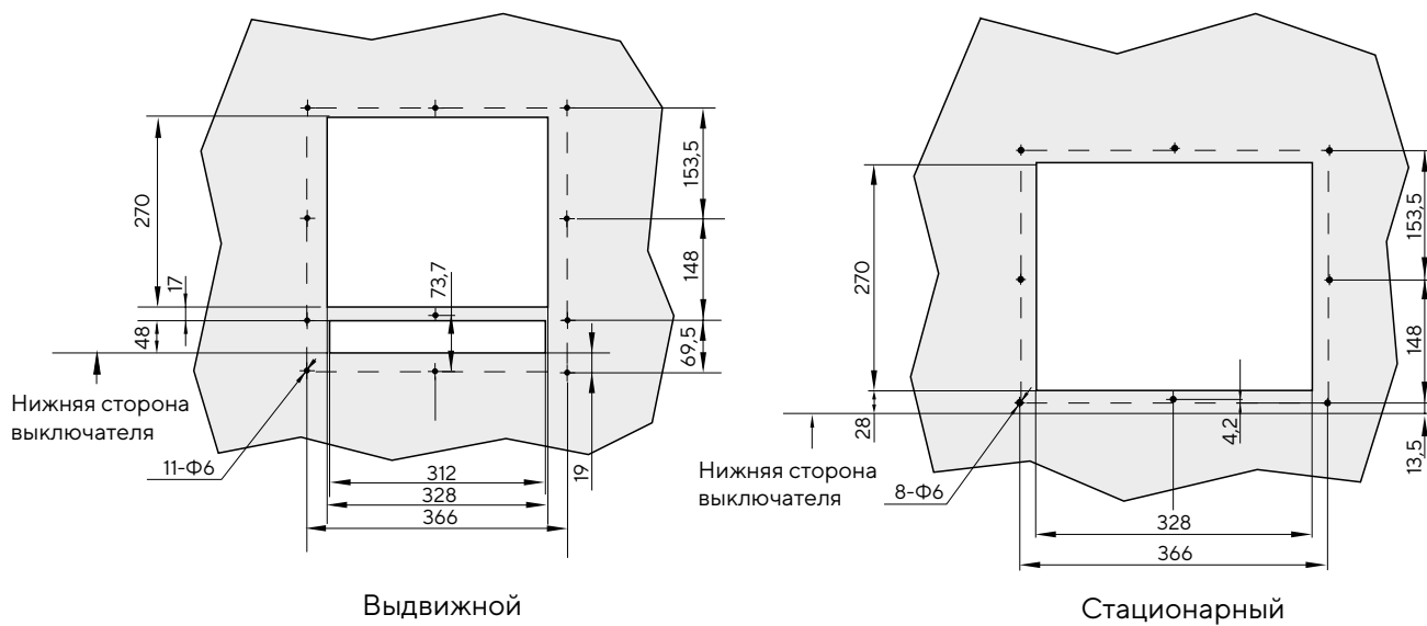
Рис. В.17. Габаритные размеры рамки обрамления выреза в двери для выключателей типоразмера F
