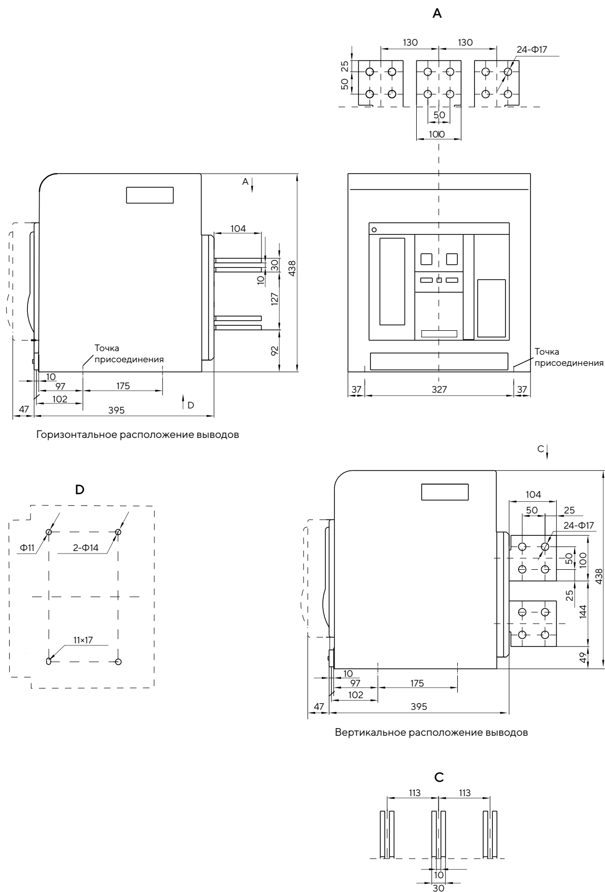
Рис. В.11. Габаритные размеры выдвижных трехполюсных выключателей типоразмера F (2500~4000 А)
